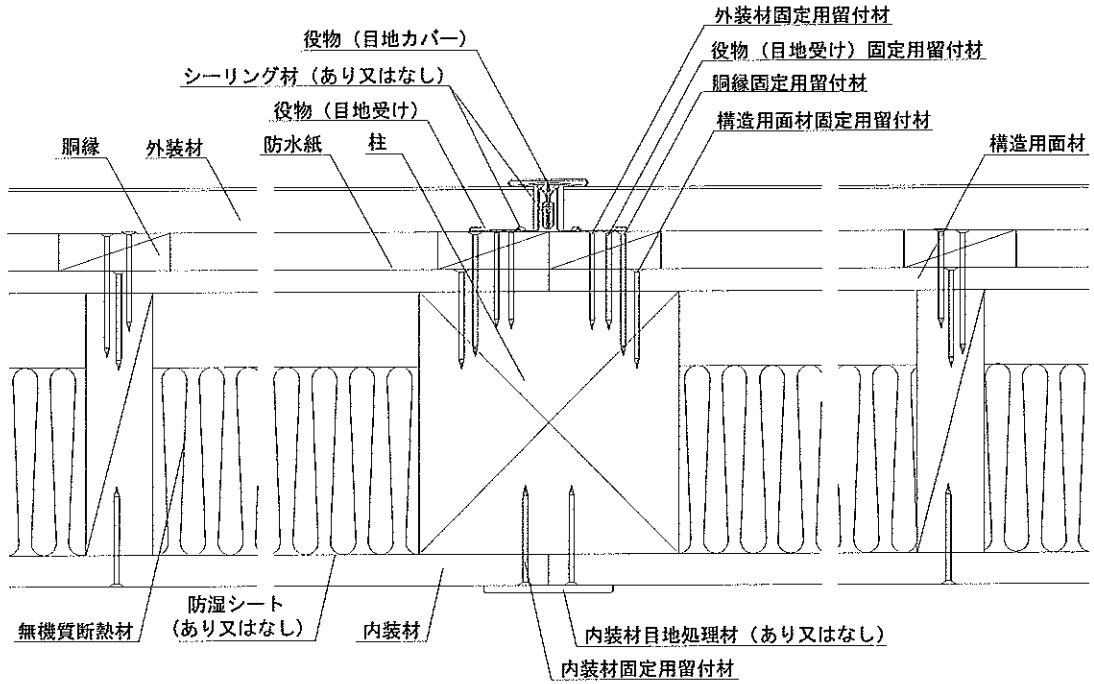
水平断面図
