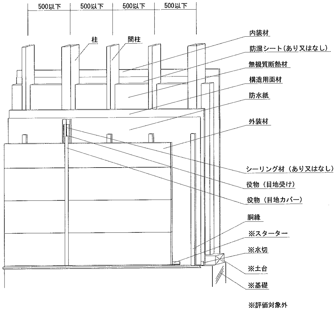
透視図
