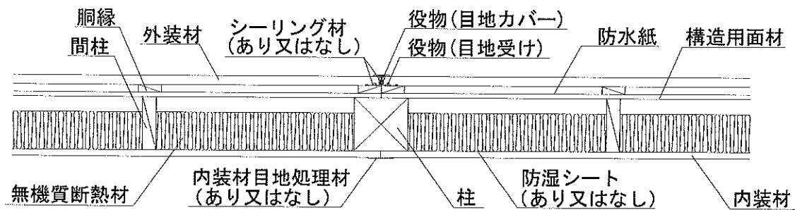
水平断面図
