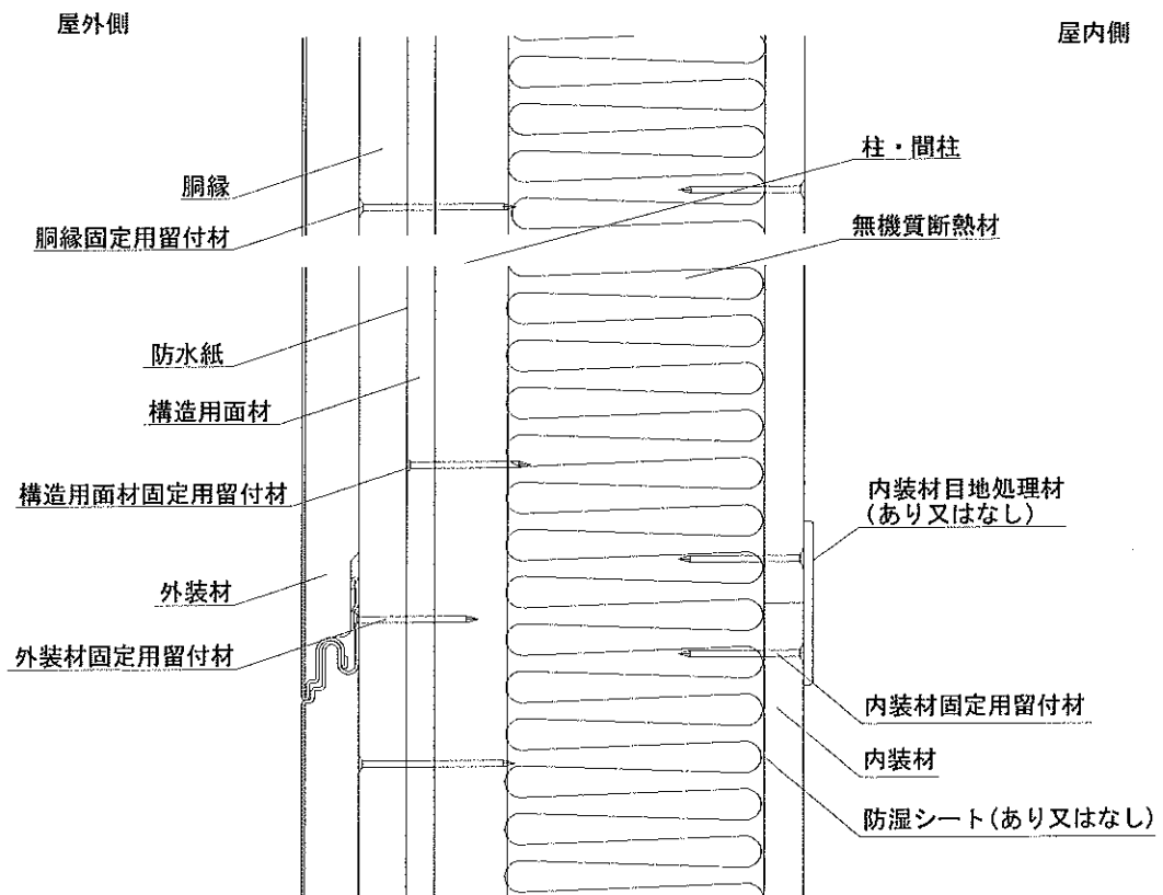
鉛直断面図
