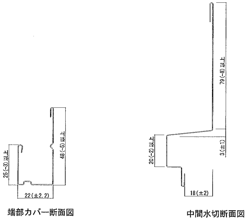
役物形状図
