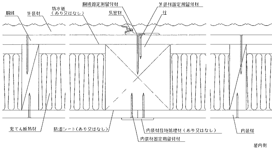
水平断面図
