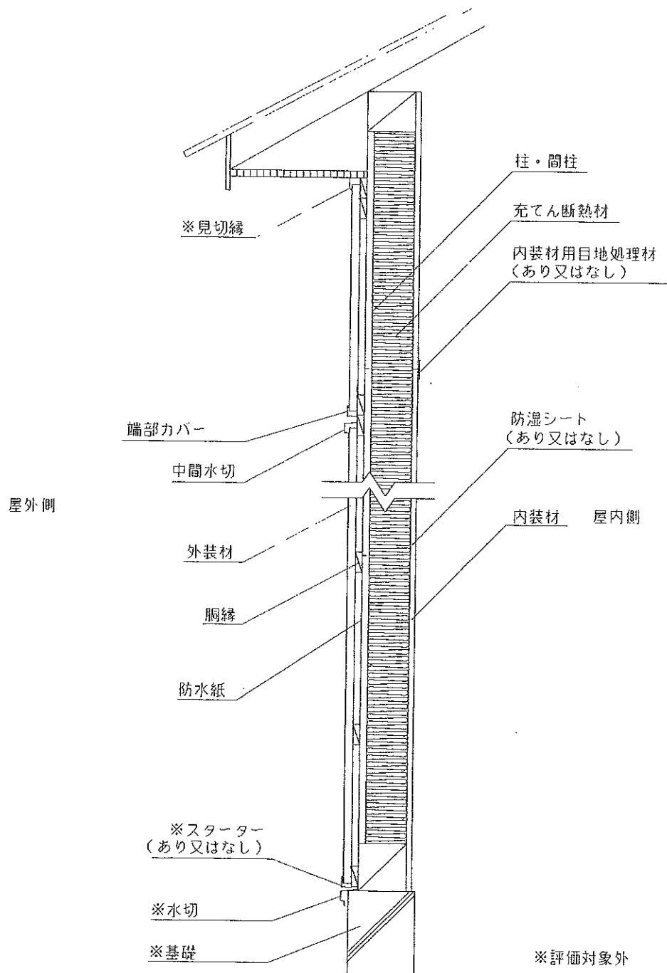
図4 施工図
