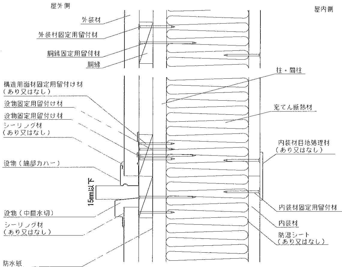
鉛直断面図
