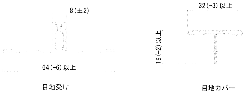
役物形状図
