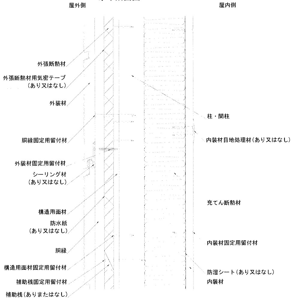
鉛直断面図
