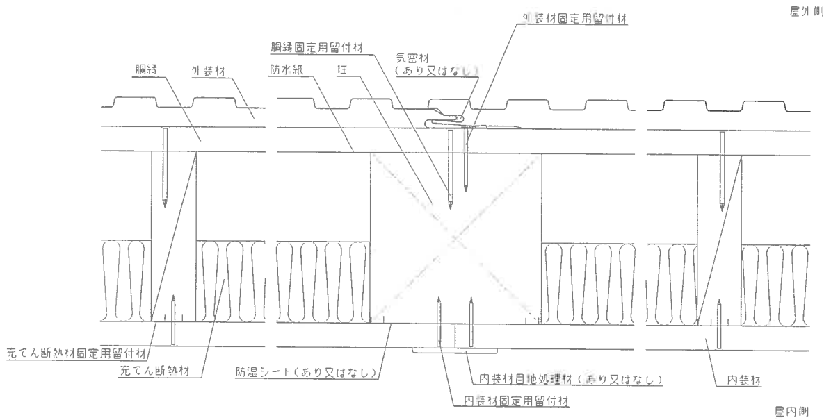
水平断面図
