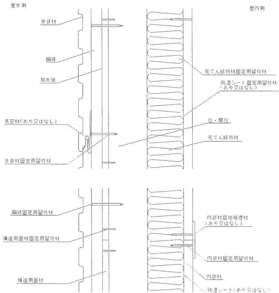
鉛直断面図
