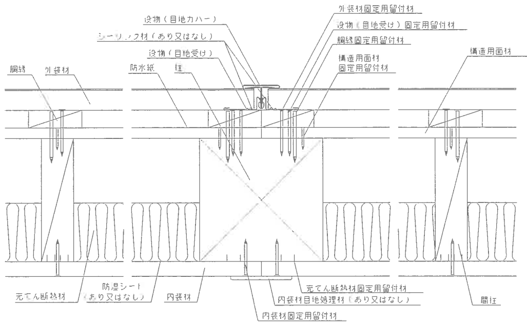
水平断面図
