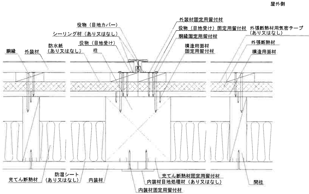
水平断面図
