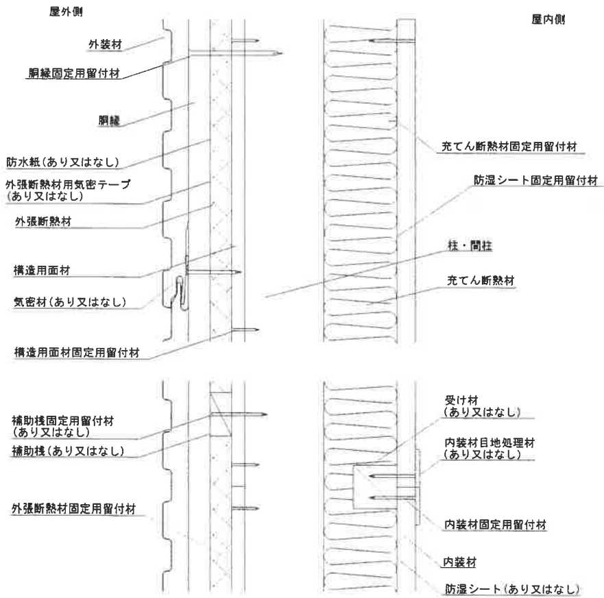
鉛直断面図
