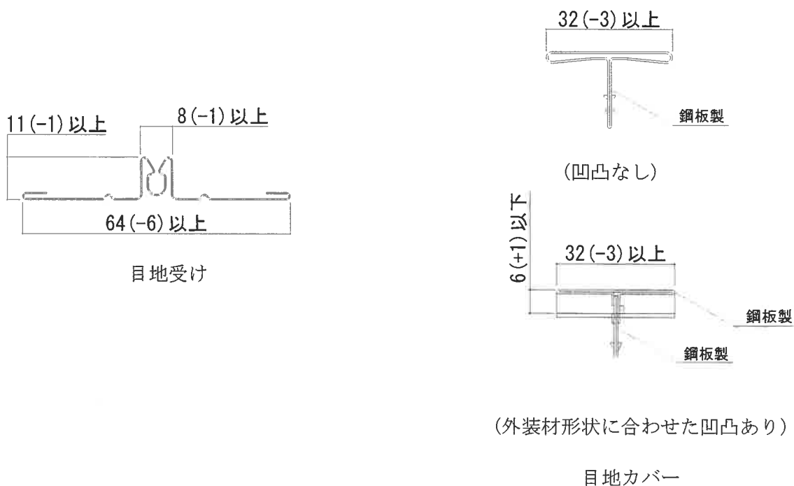
役物断面形状図
