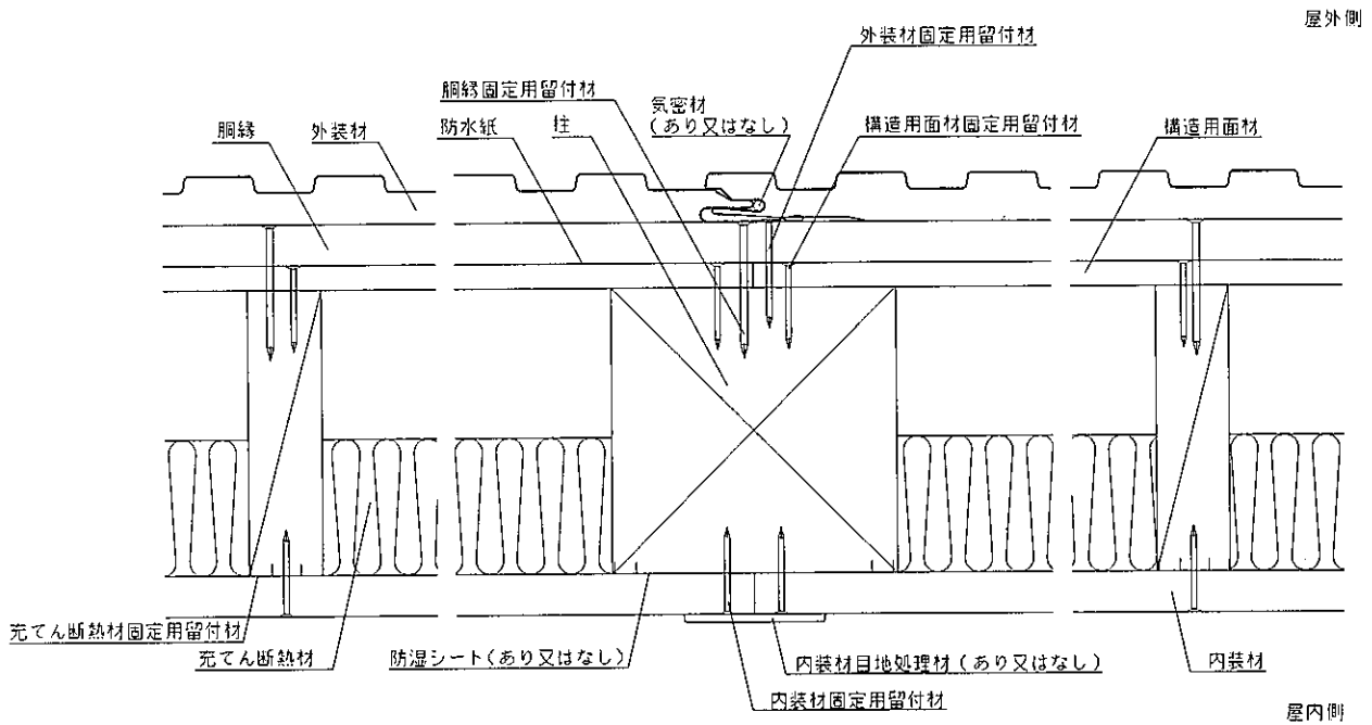
水平断面図
