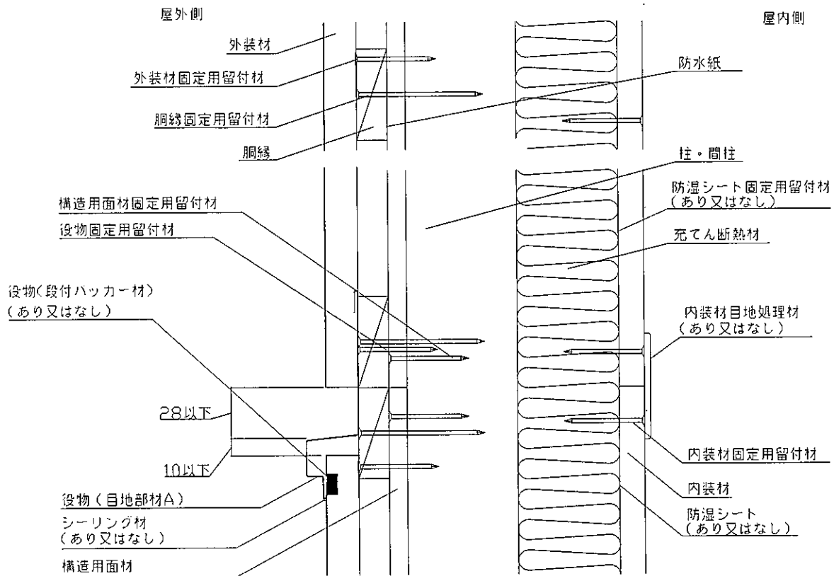
鉛直断面図(目地部材Aのみ)
