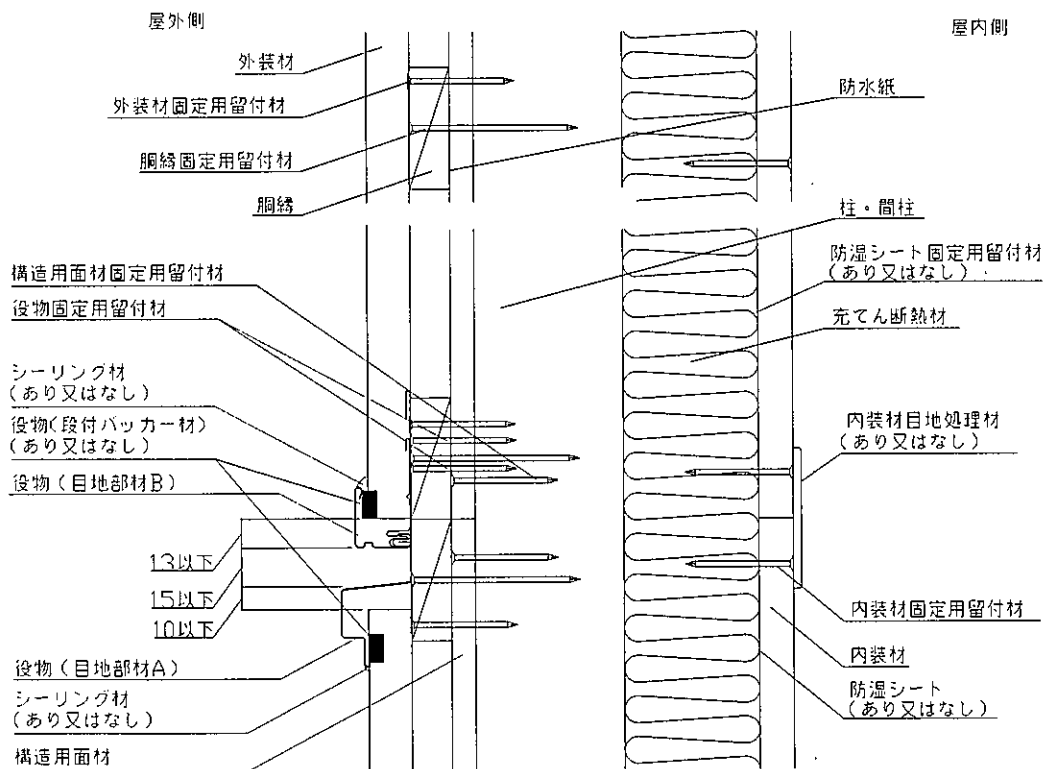
鉛直断面図(目地部材B 2ピースタイプ)
