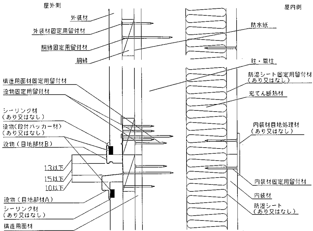
鉛直断面図(目地部材B 1ピースタイプ)
