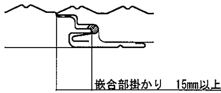
嵌合部詳細
