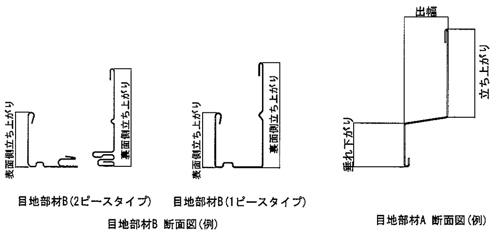
図5 構造説明図
