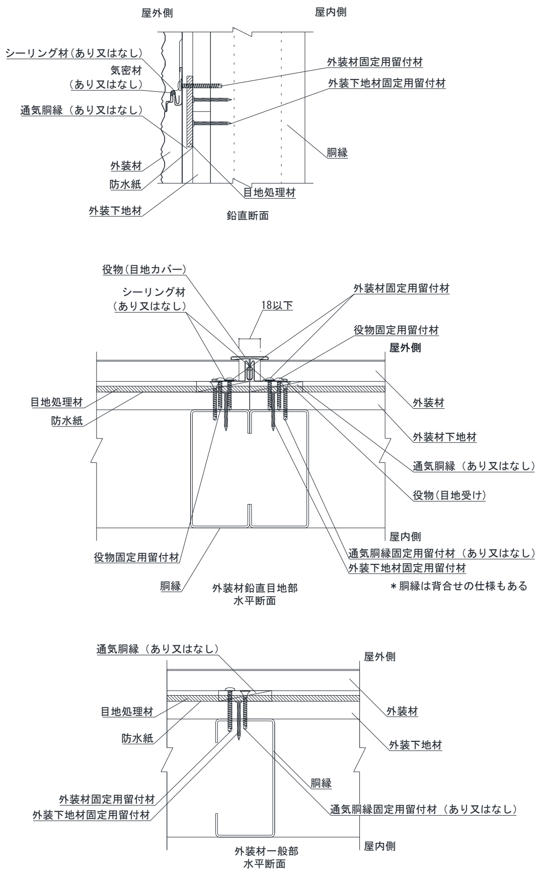
図2 構造説明図 (胴縁が軽量形鋼の場合)
