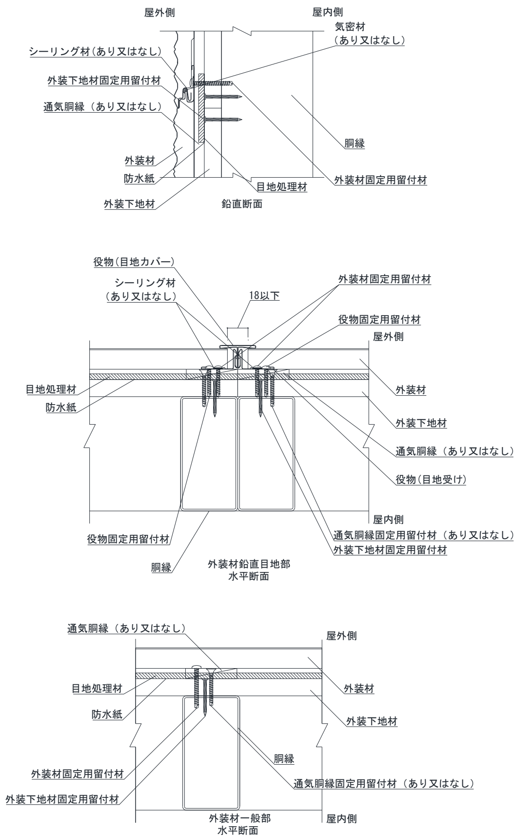
図4 構造説明図 (角縁が一般構造用角形鋼管の場合)
