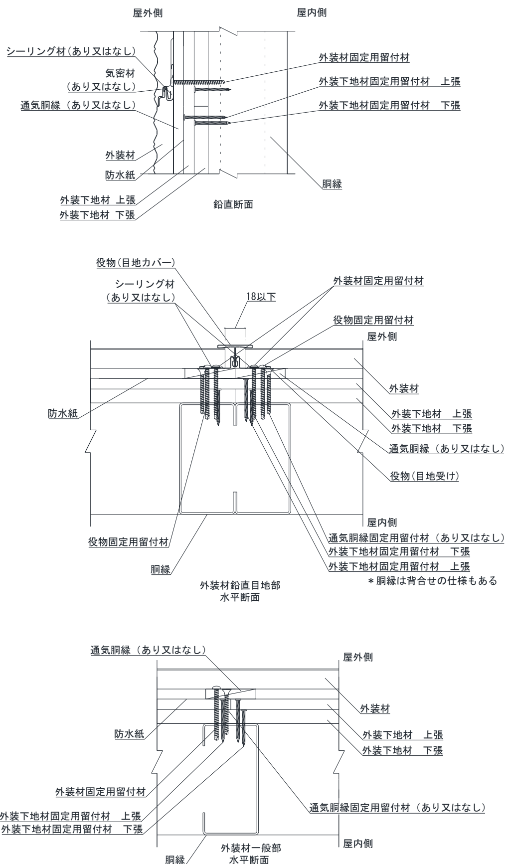
図2 構造説明図 (胴縁が軽量形鋼・外装下地材重張りの場合)
