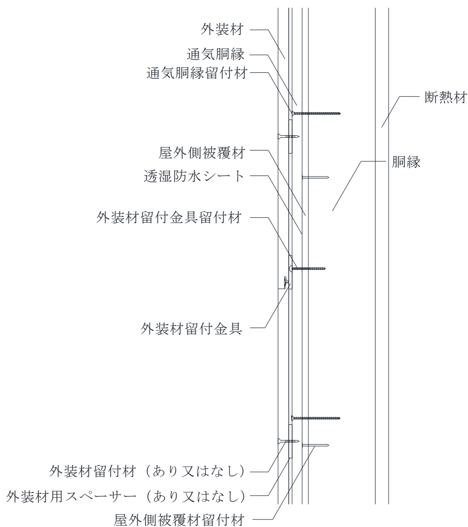
断面図
