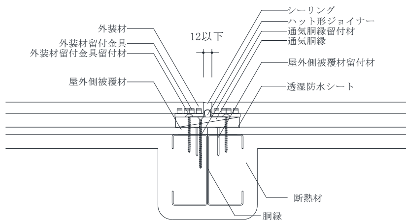
平面图
