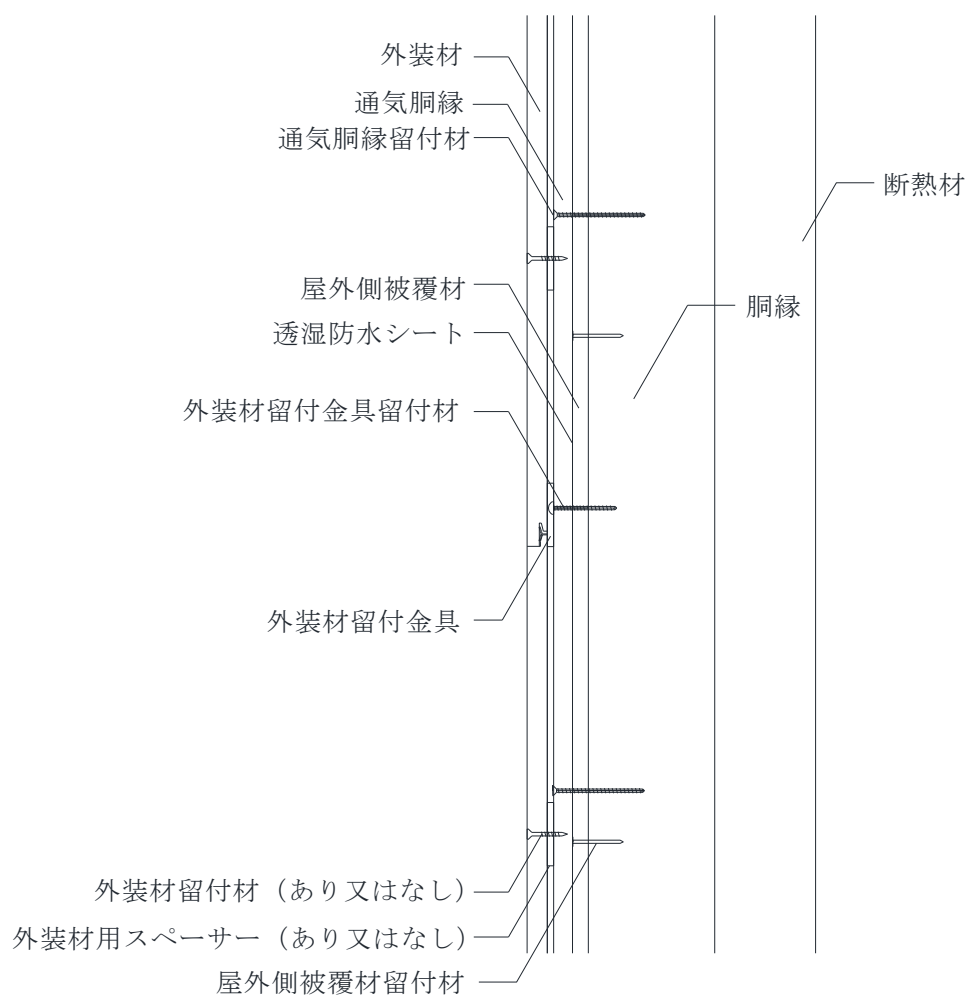
平面図
