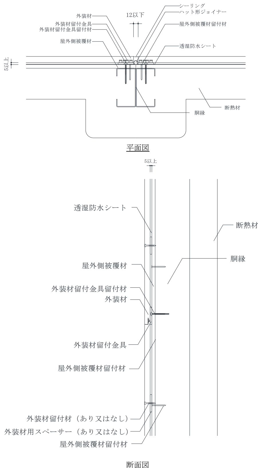
図7 構造説明図（通気胴縁なし仕様）断熱材最厚
