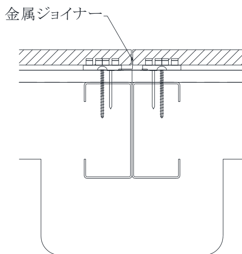
②金属ジョイナー目地
