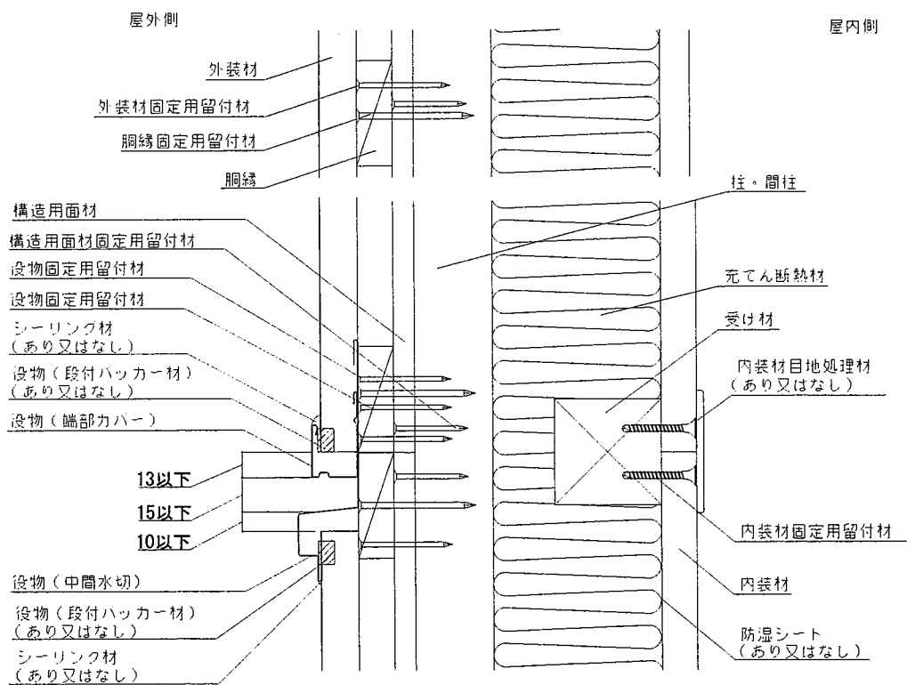
鉛直断面図
