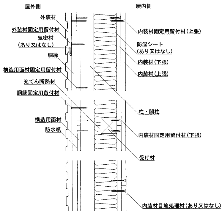
鉛直断面図
