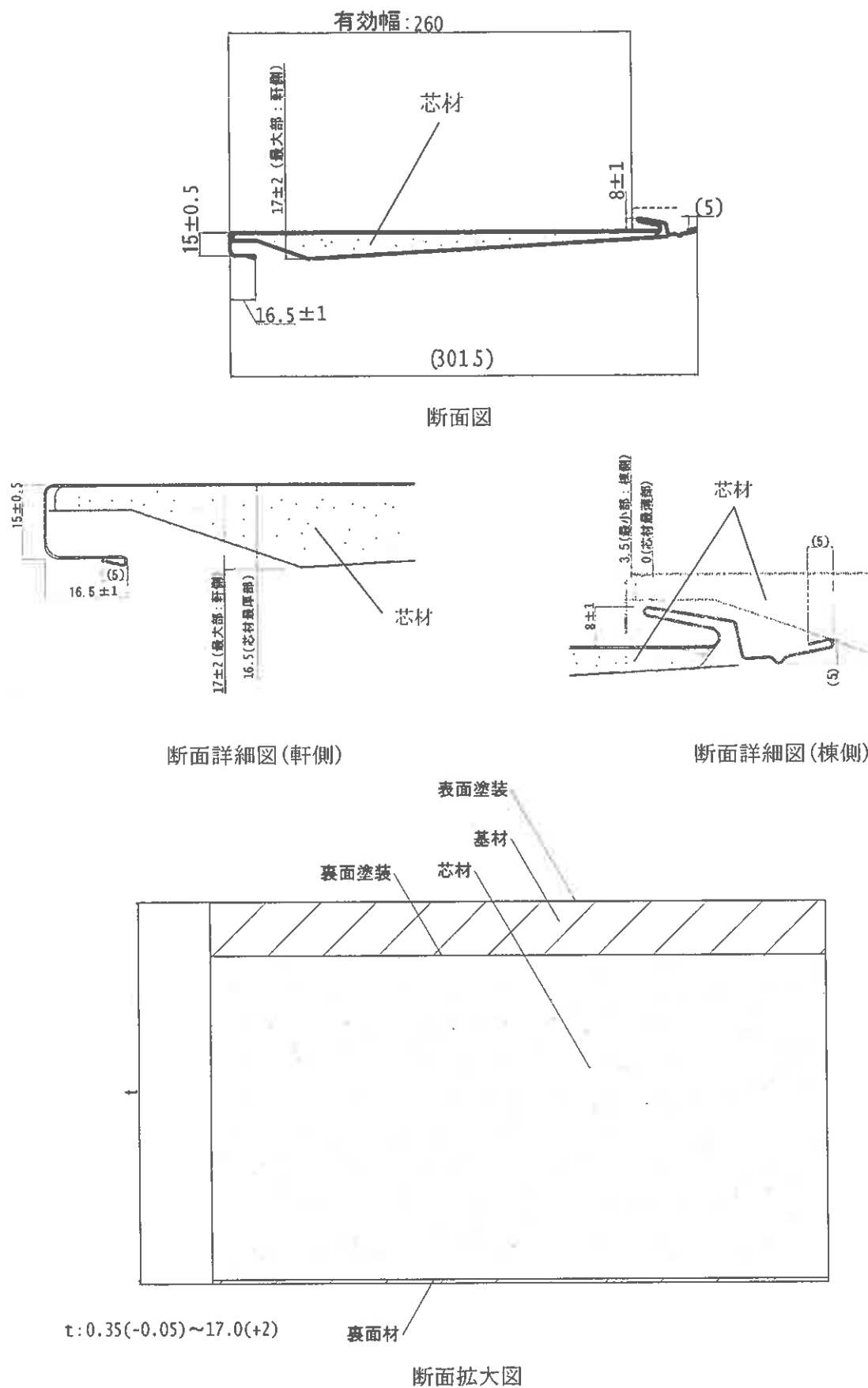
図2 構造説明図
