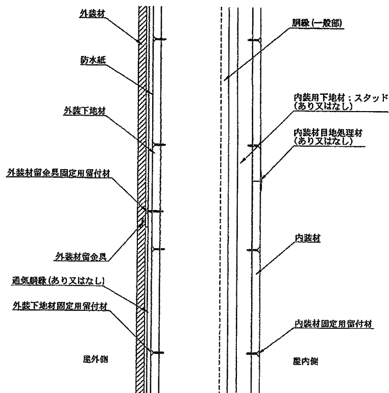
鉛直断面図
