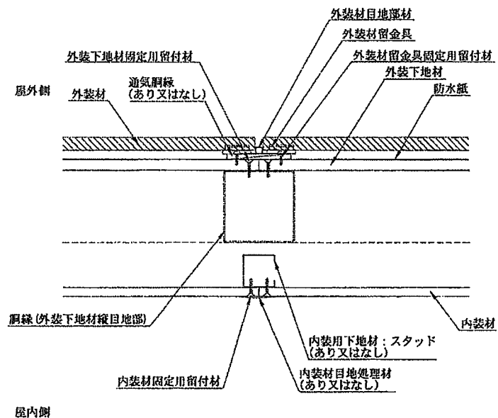
水平断面図
