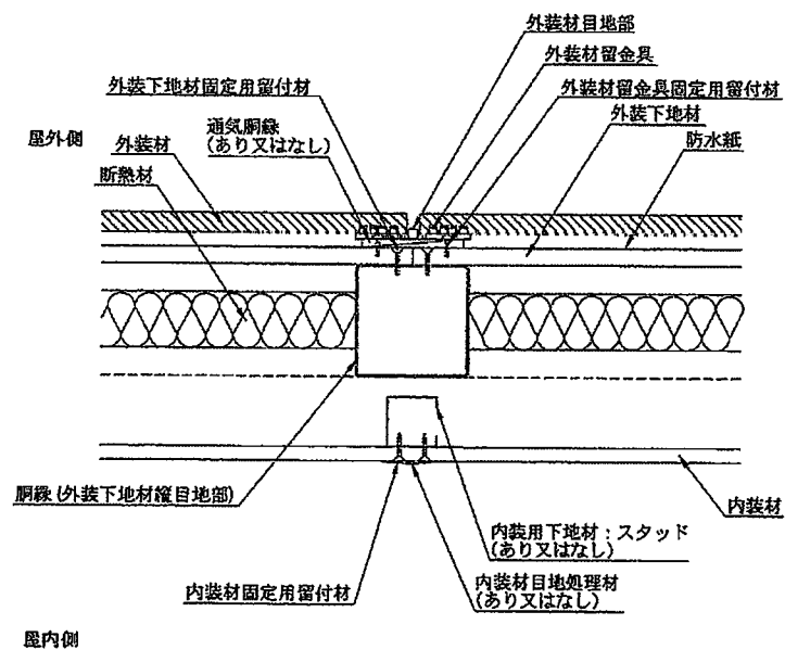
水平断面図
