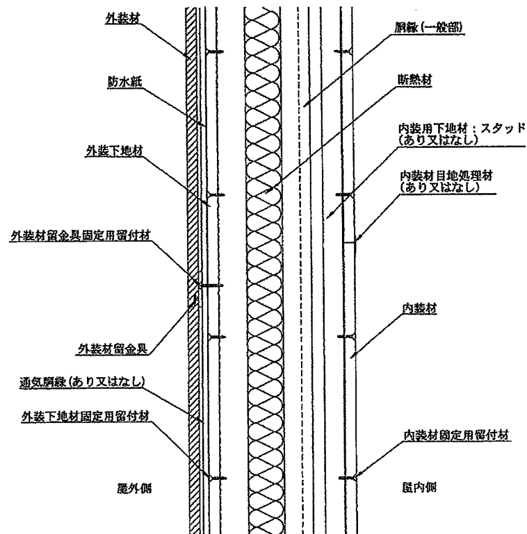
鉛直断面図
