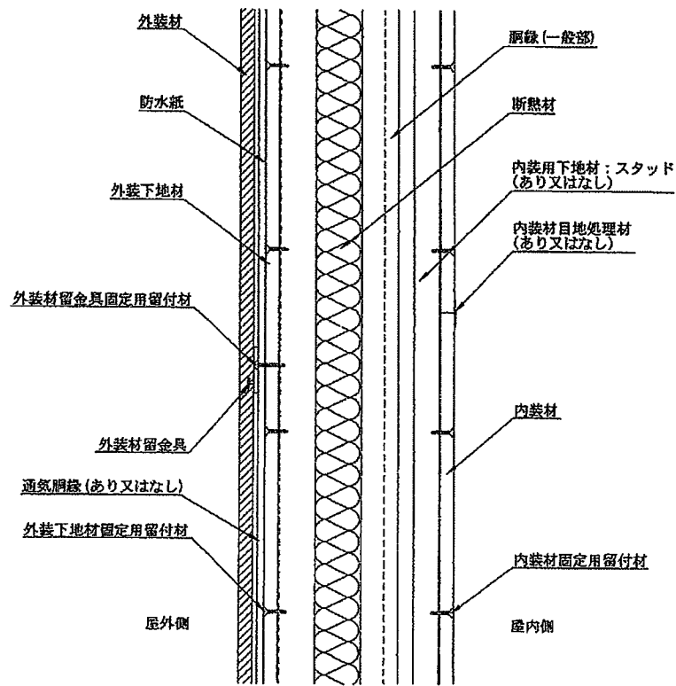
鉛直断面図
