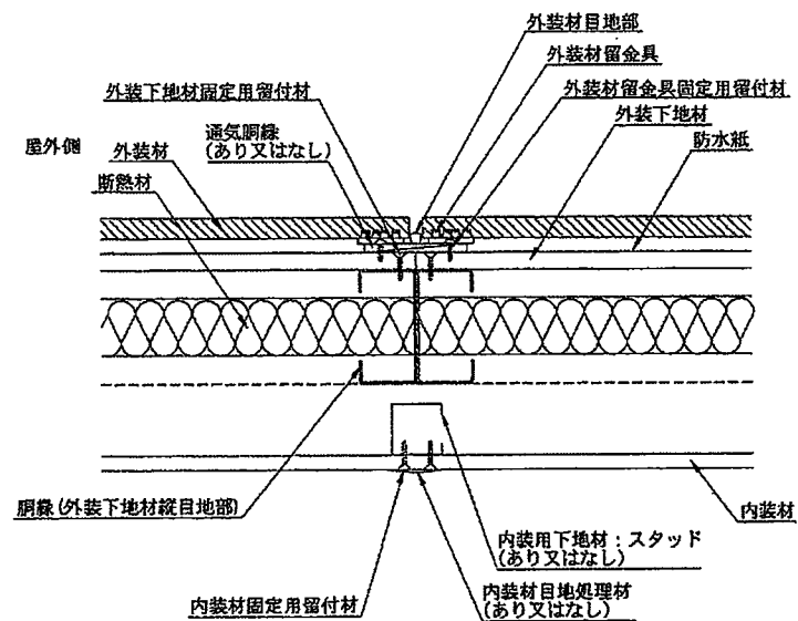
水平断面図
