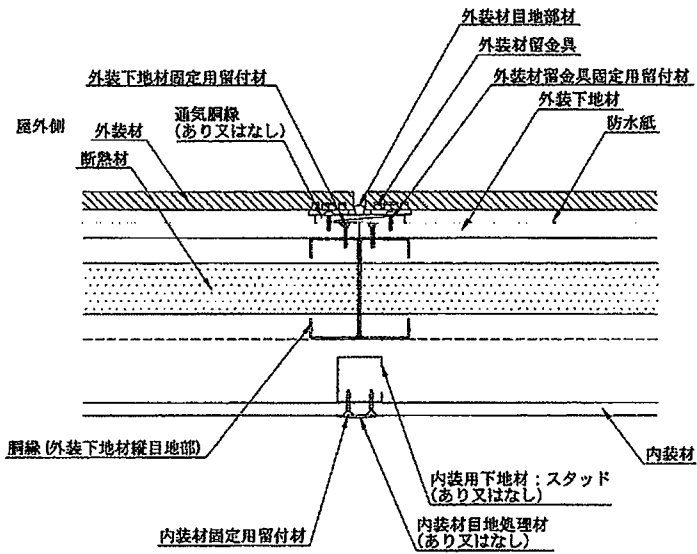
水平断面図
