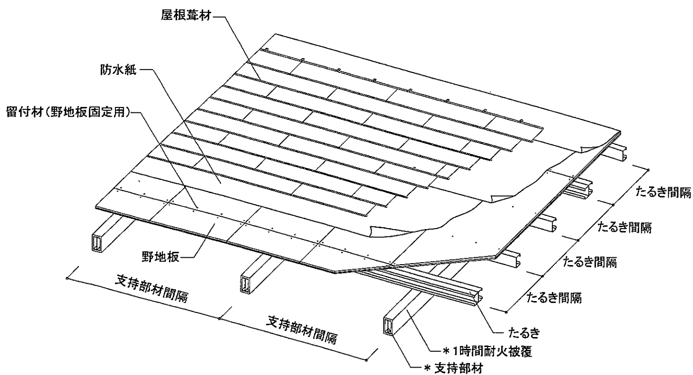
透視図(横葺、連続支持)
