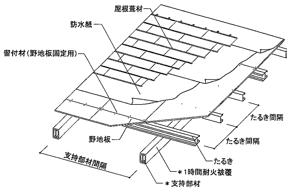
透視図(平葦、単純支持)
