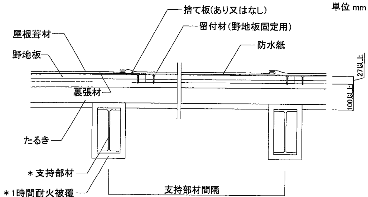
A-A断面詳細図(平葺)
