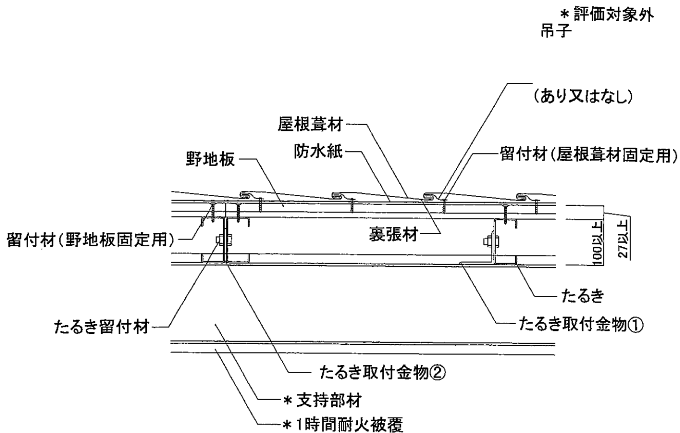
A-A断面詳細図(横葺)
