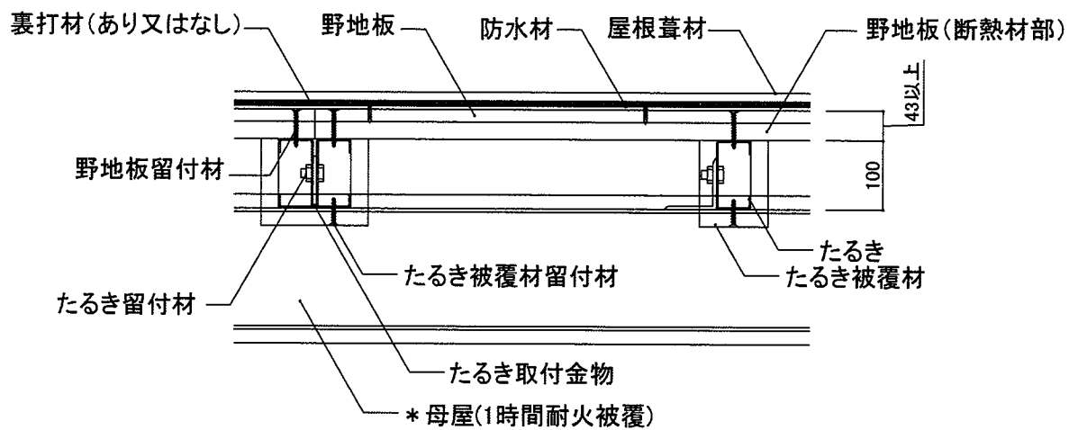
図4 構造説明図(2) たて平葺き仕様
