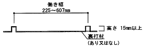
畳材断面(代表的な仕様)
