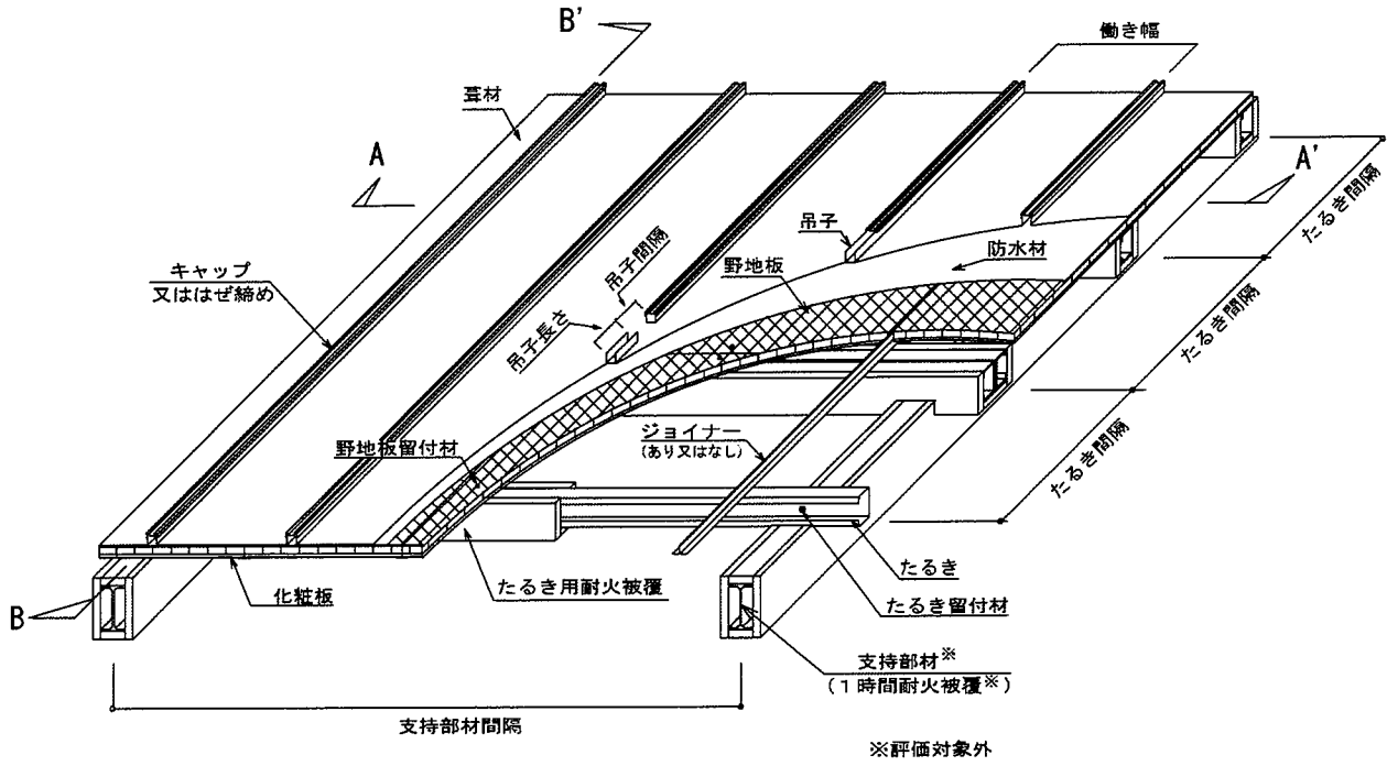
透視図
