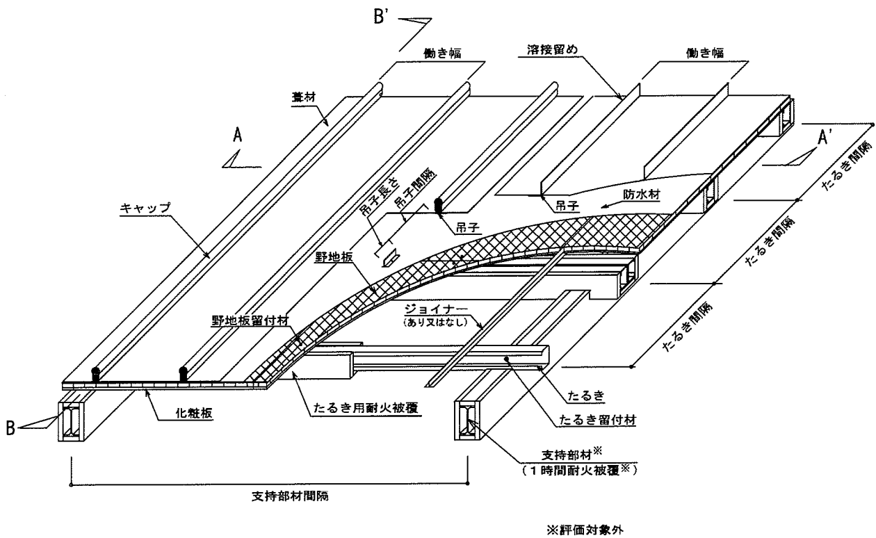
透視図
