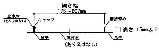
葺材断面 (代表的な仕様)
