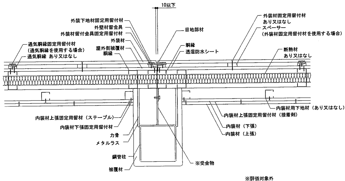
図2 構造説明図
