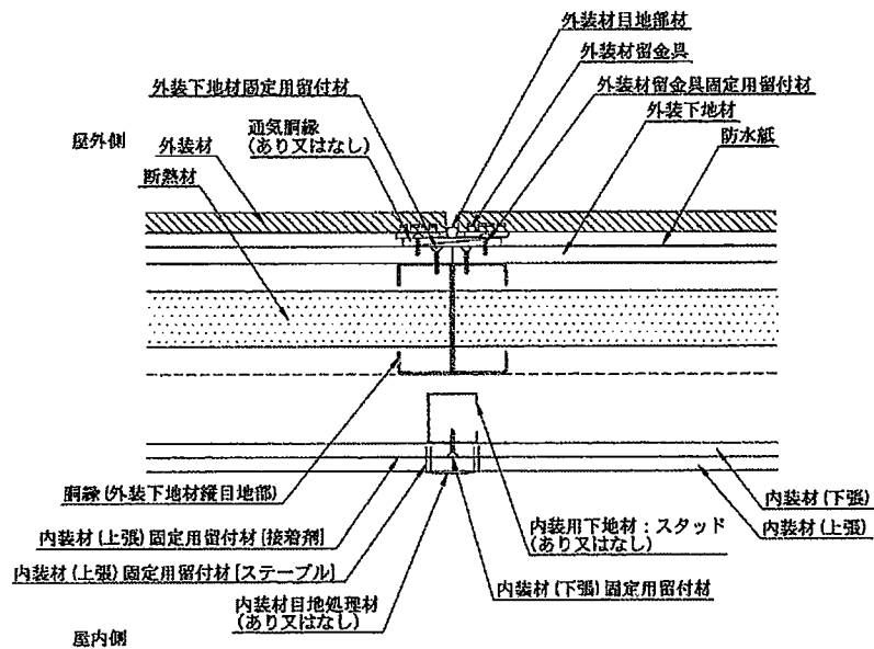
水平断面図
