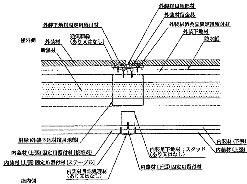
水平断面図
