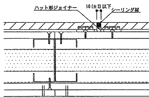
②ハット形ジョイナーとシーリング材の併用目地
