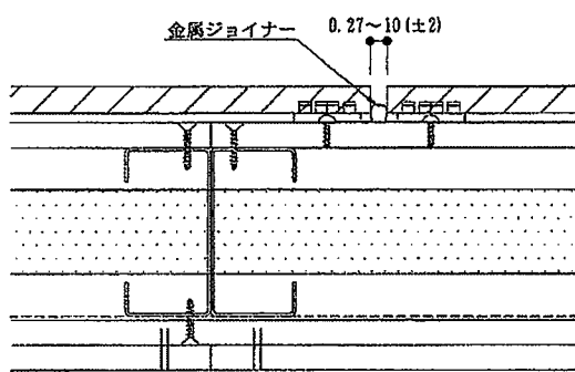
①金属ジョイナー目地
