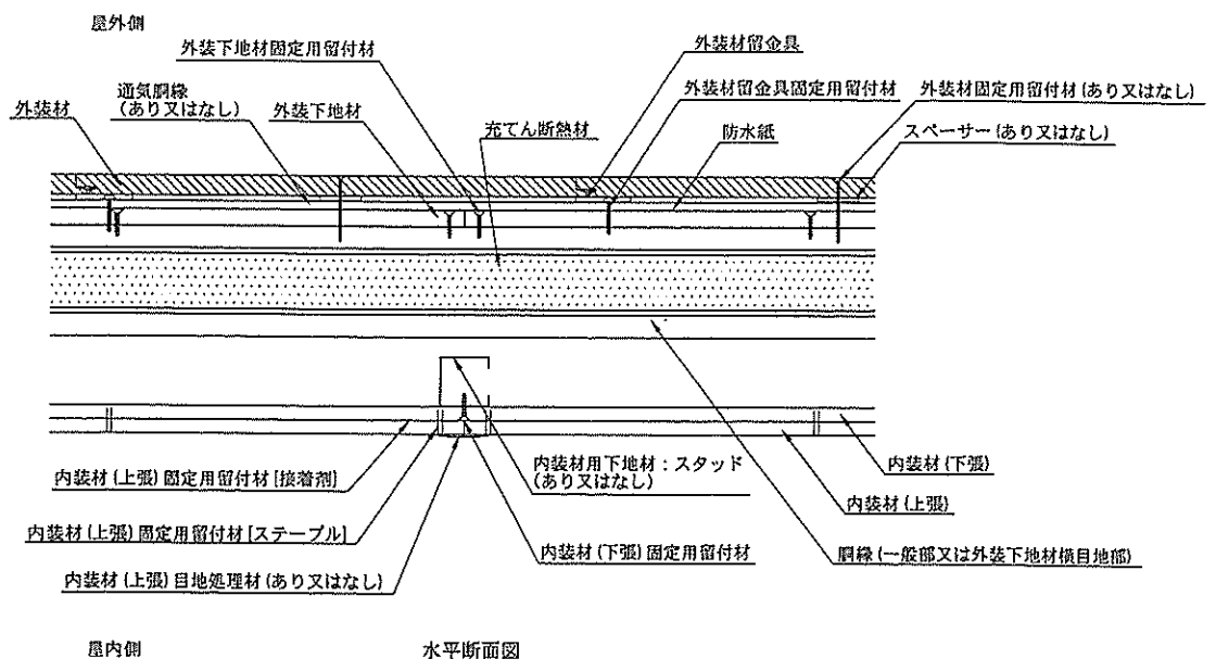
水平断面図
