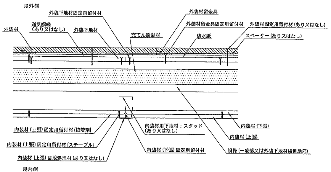
水平断面図
