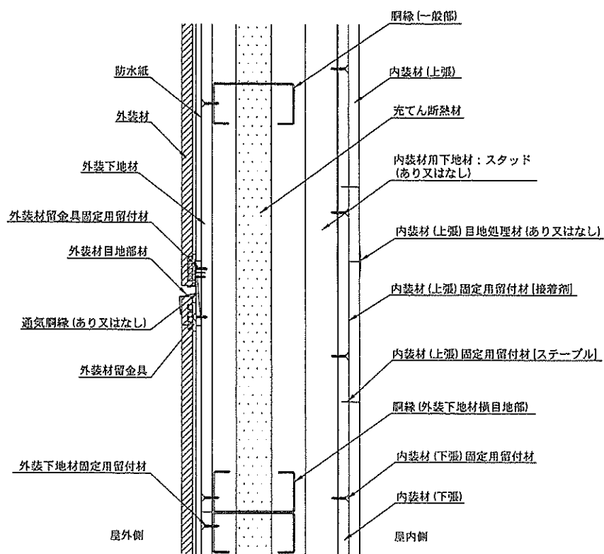
鉛直断面図
