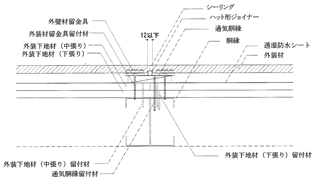
平面図
