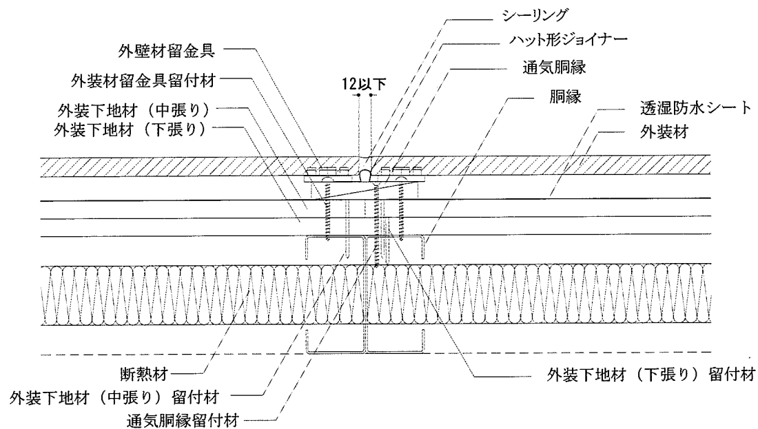
平面図
