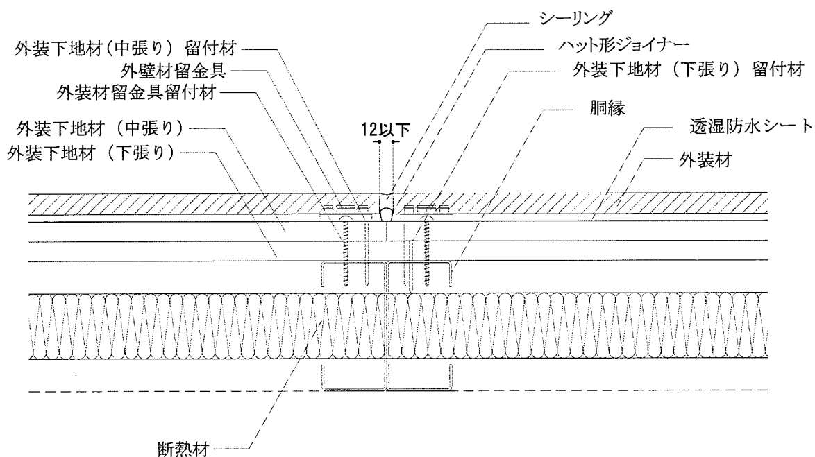
平面図
