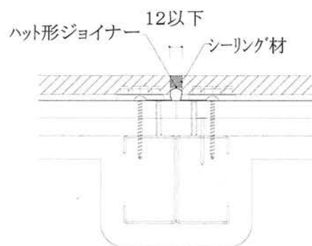
①ハット形ジョイナー＋シーリング目地
