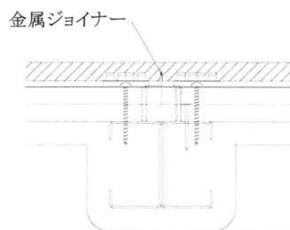
②金属ジョイナー目地
