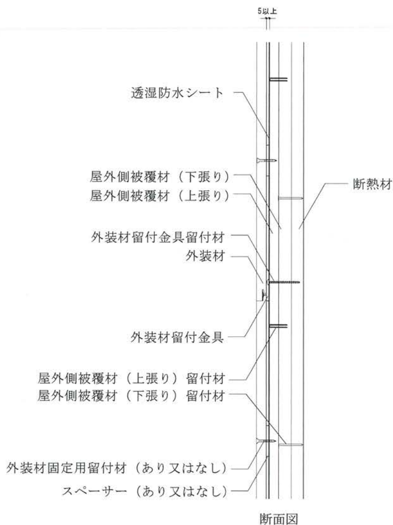
図3 構造説明図 (通気胴縁なし仕様)
