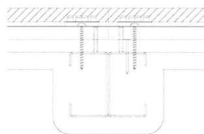
④突き付け目地
