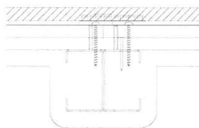
③本実・合いじゃくり目地
