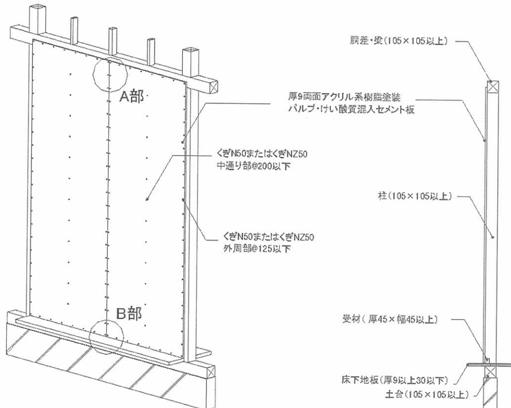
図2 施工図詳細 (mm)
