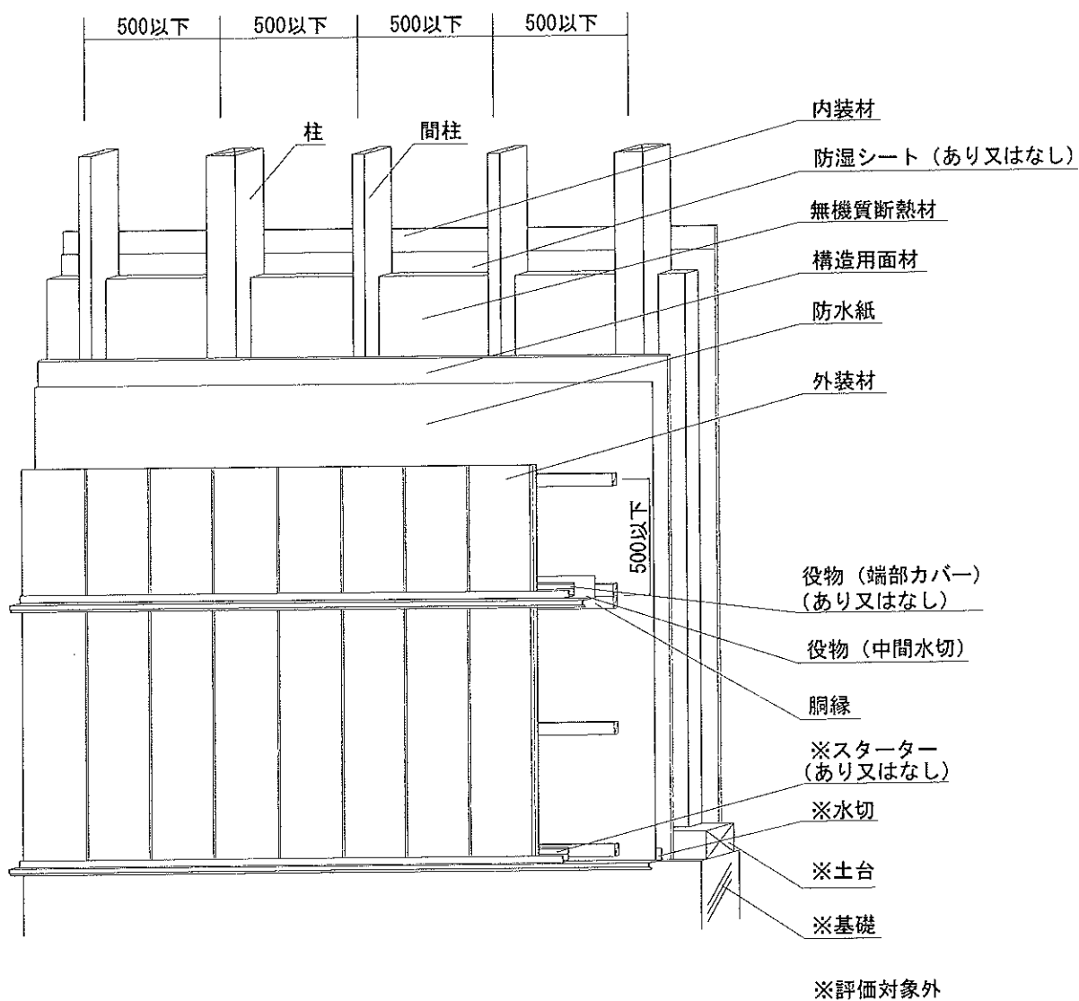
透視図
