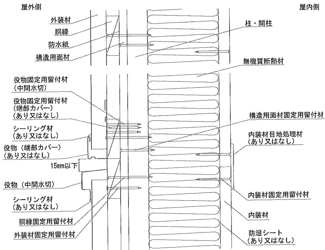
鉛直断面図
