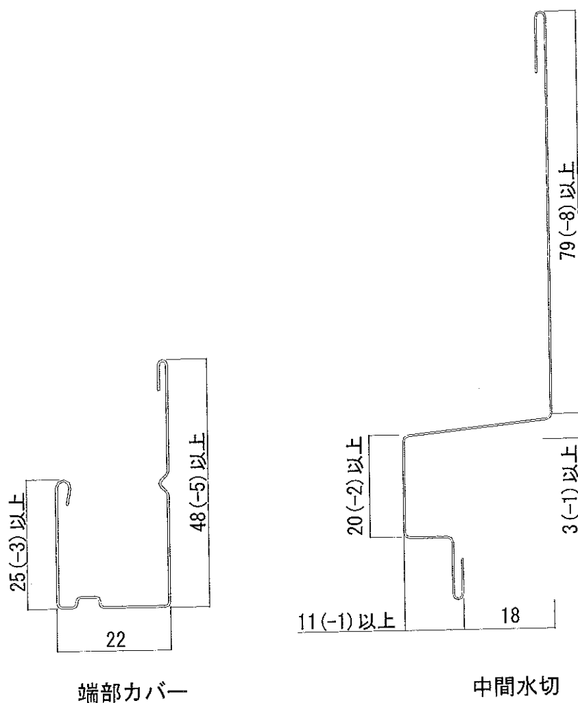
図4 役物形状図
