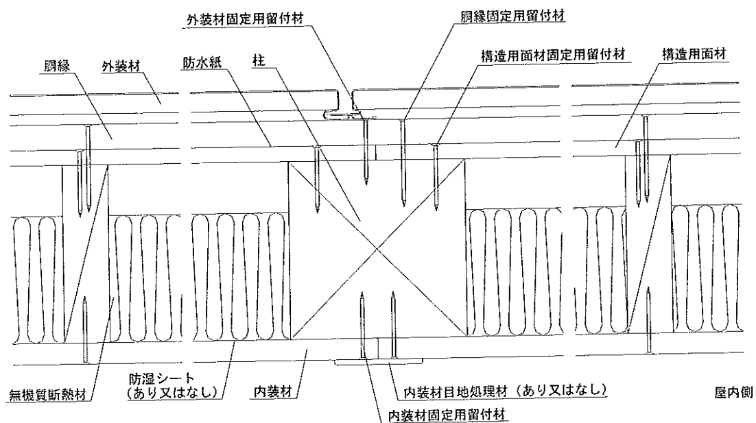
水平断面図
