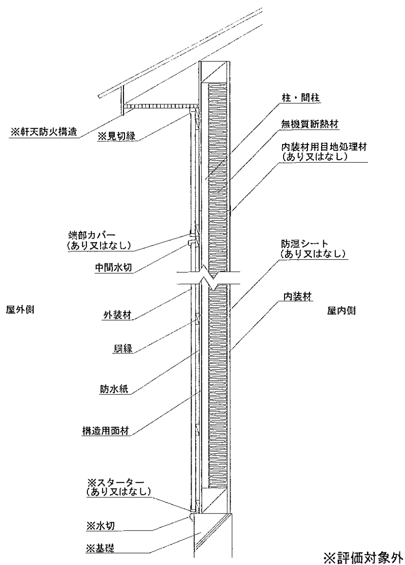
鉛直断面図
