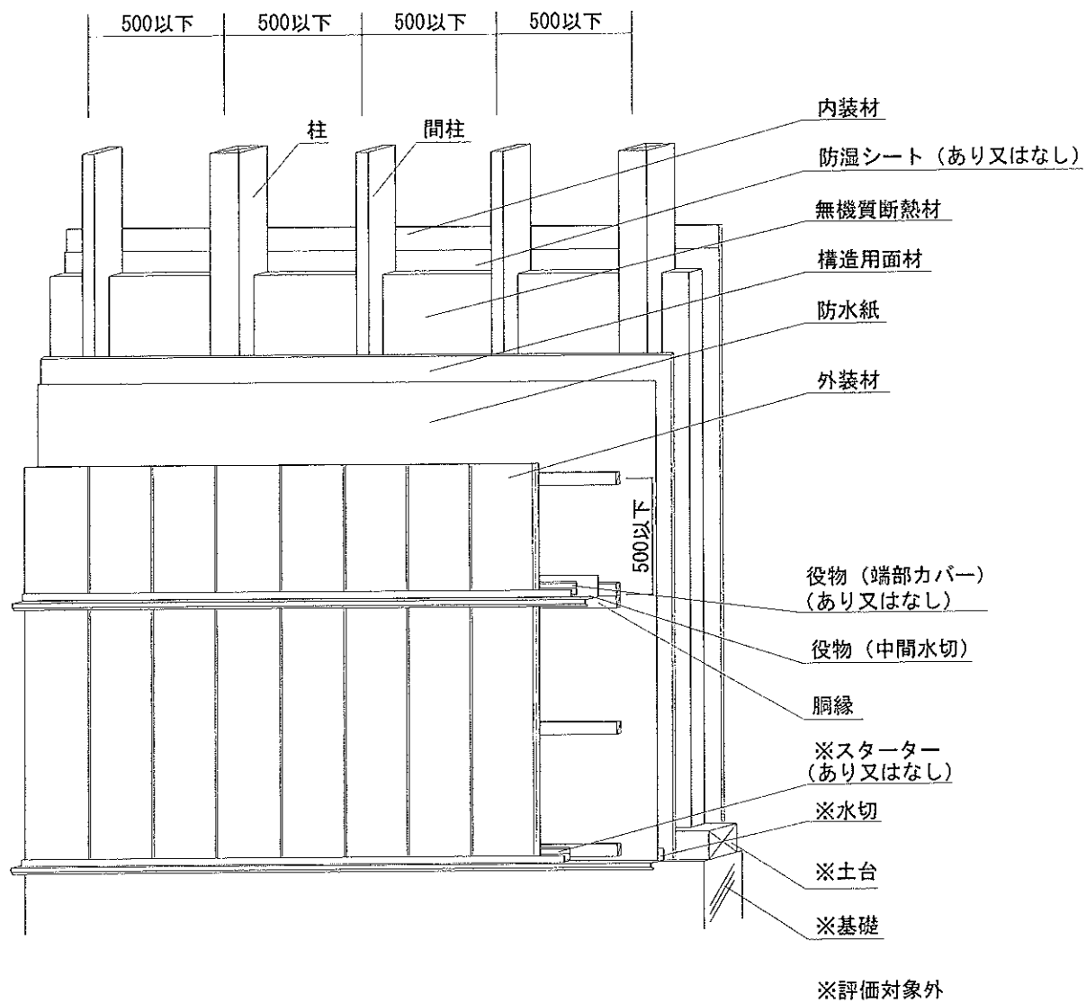
透視図
