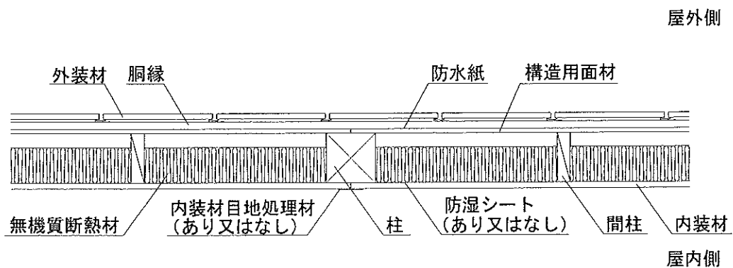
水平断面図
