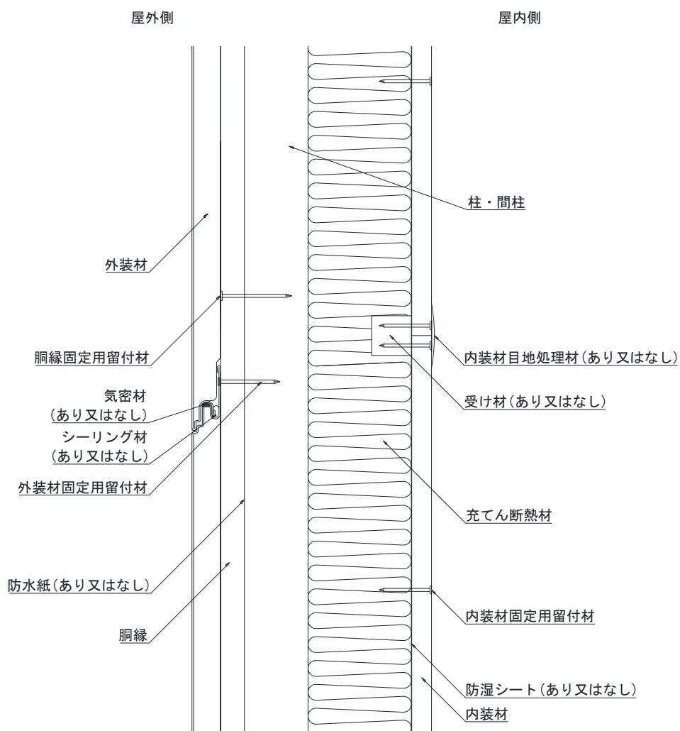
鉛直断面図
