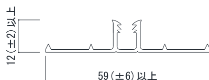
目地受け(樹脂製)
