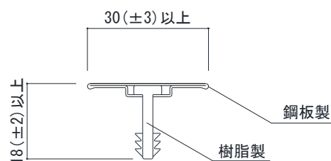
目地カバー(鋼板製及び樹脂製)
