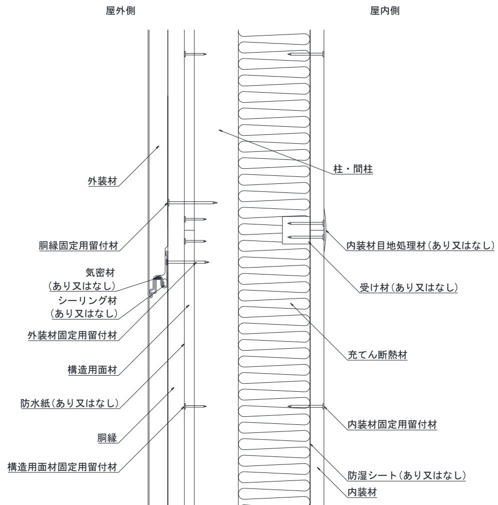
鉛直断面図
