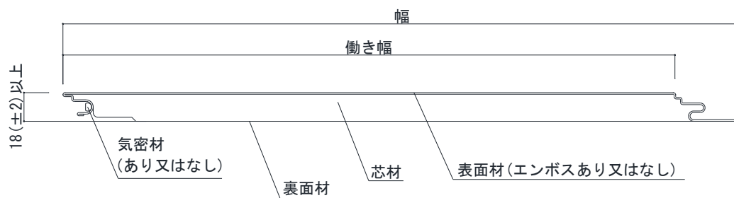
外装材断面図
