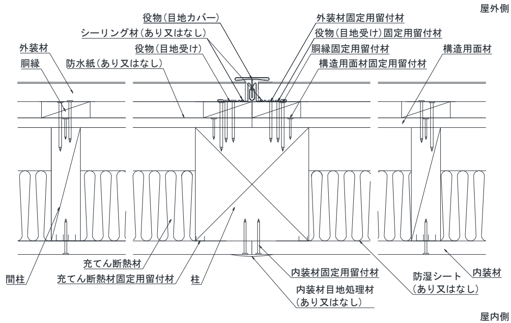
水平断面図
