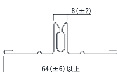
目地受け(鋼板製)
