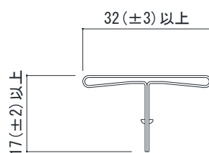
目地カバー(鋼板製)
