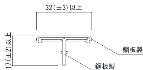
目地カバー(鋼板製)
