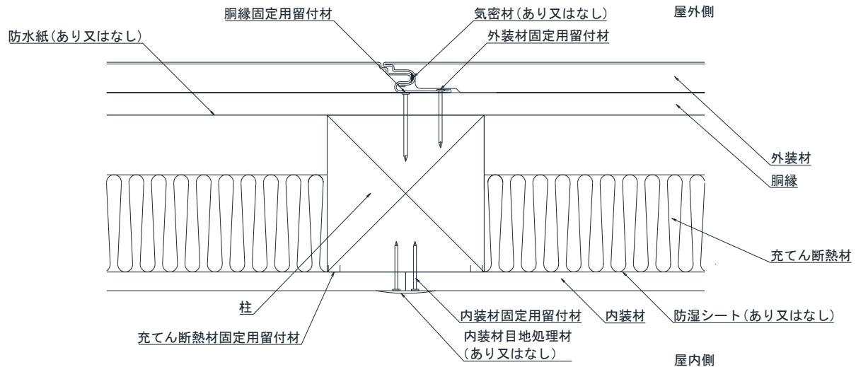
水平断面図
