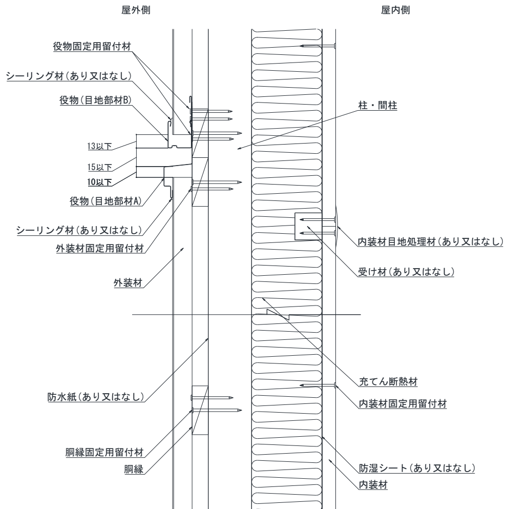
水平断面図
