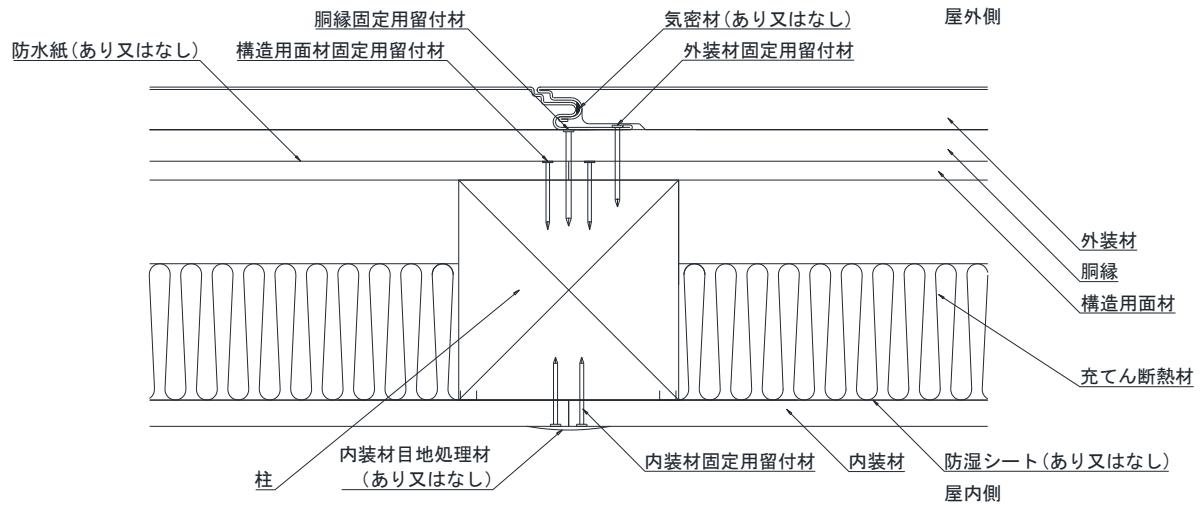
水平断面図
