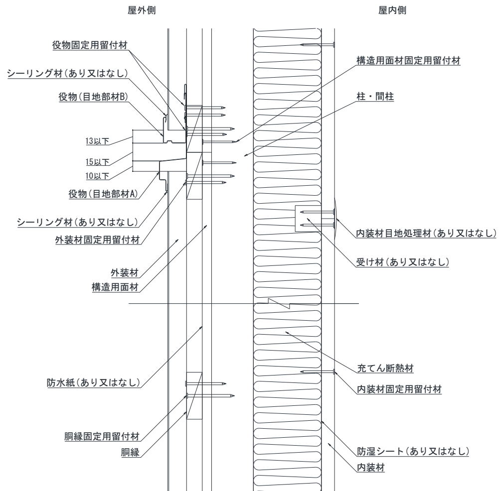
鉛直断面図
