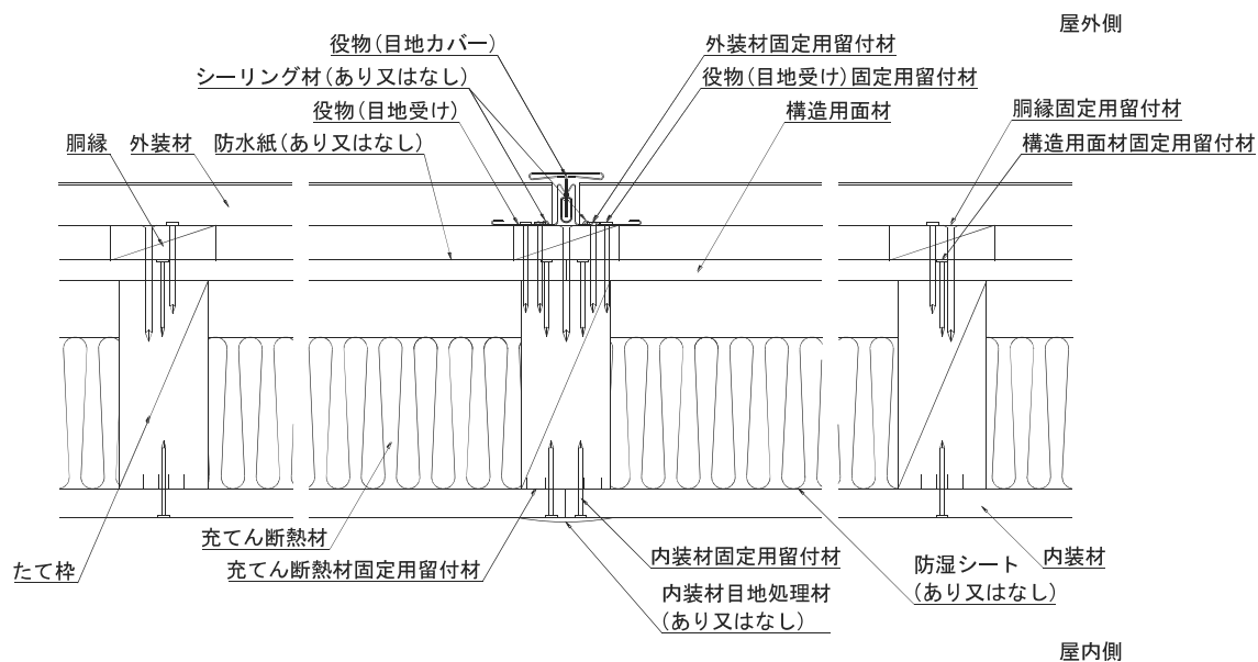
水平断面図
