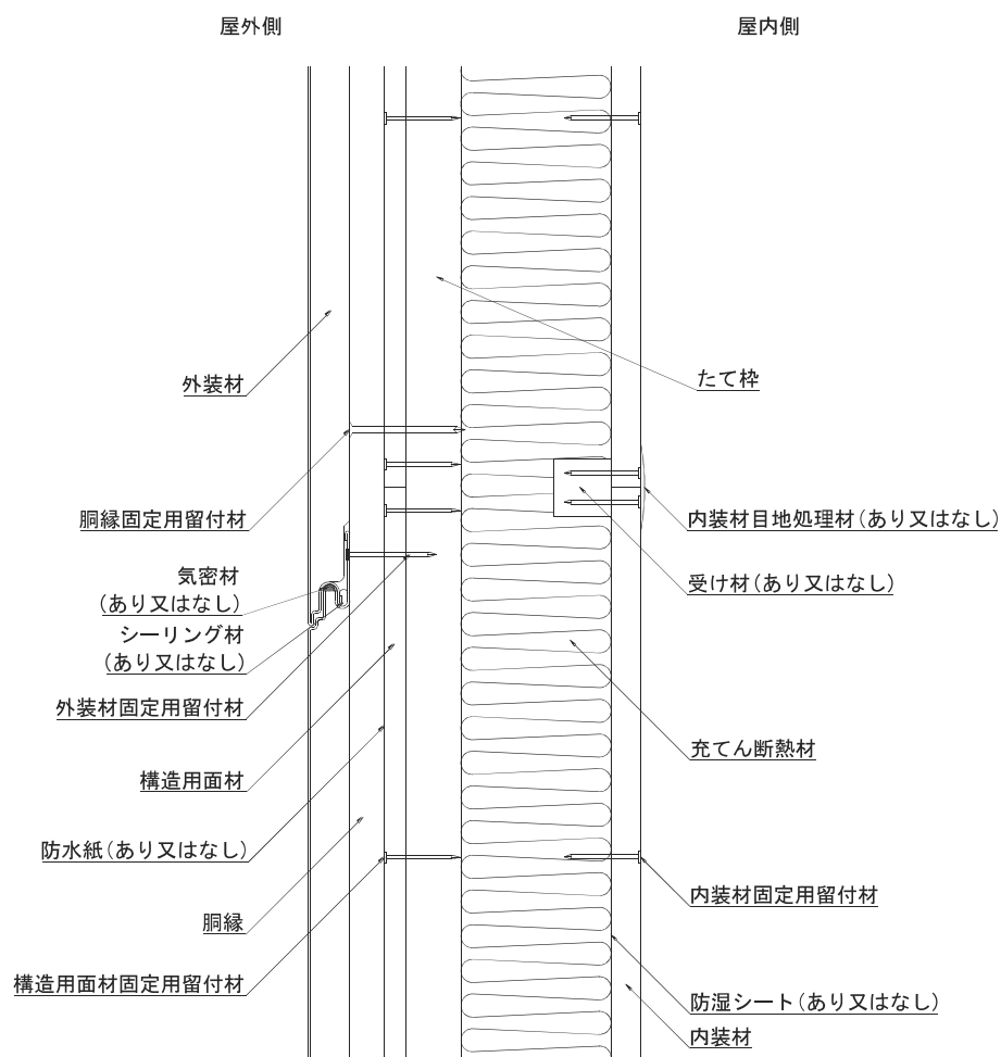
水平断面図
