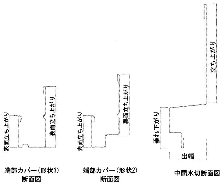
役物形状図
