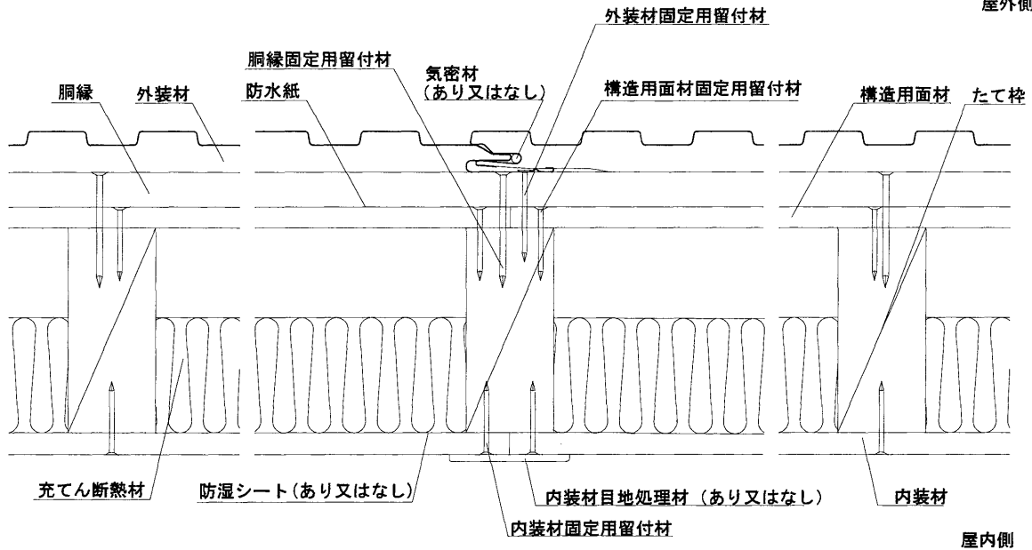
水平断面図
