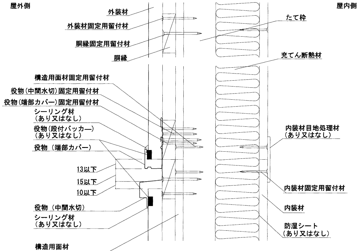
鉛直断面図
