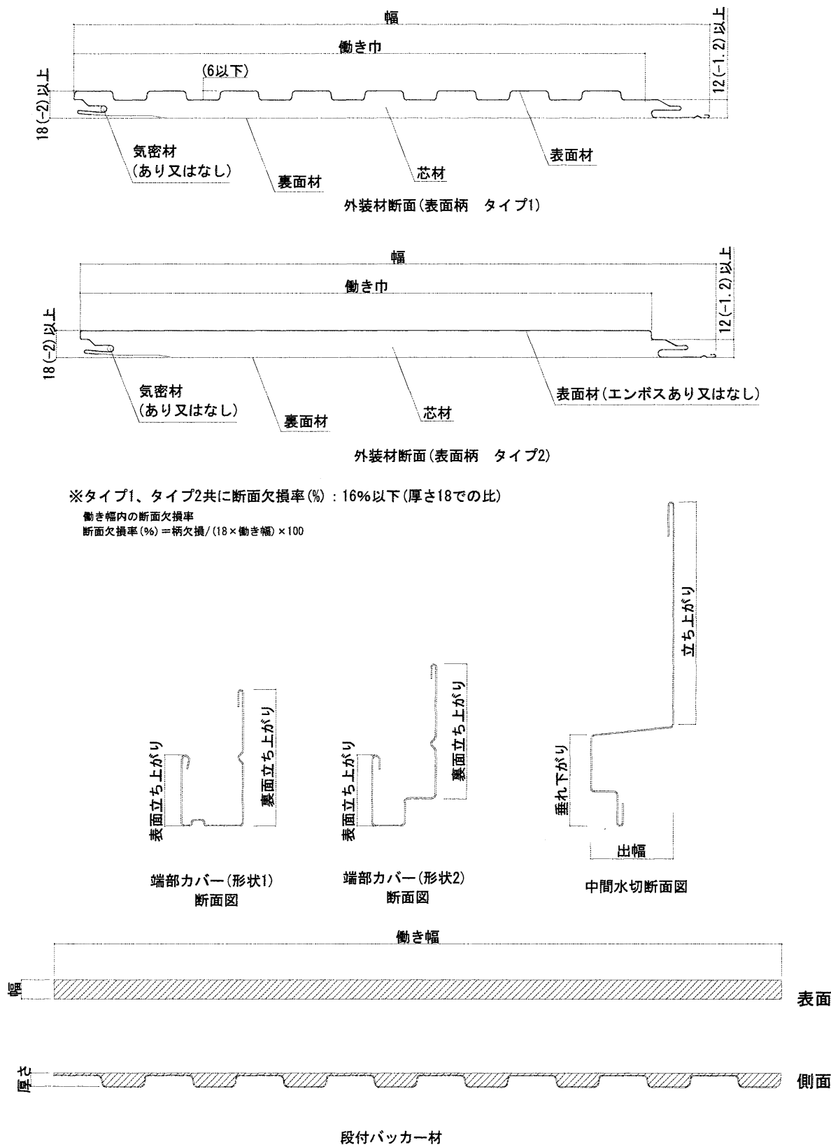
図 3 構造説明図
