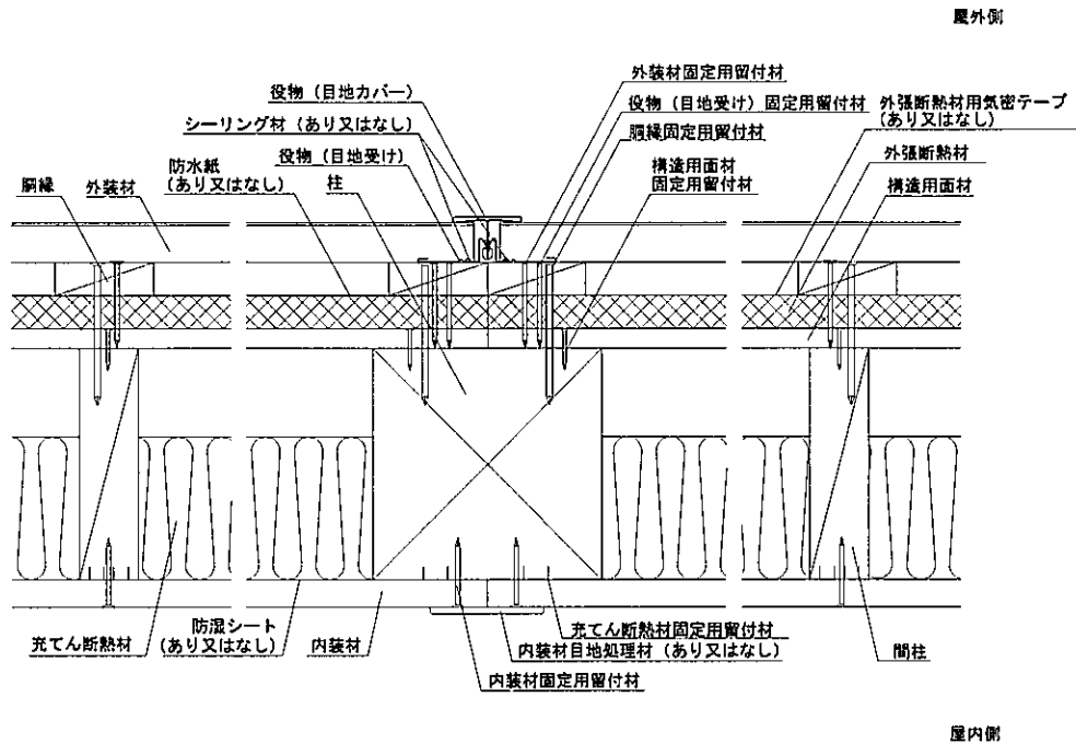
水平断面図
