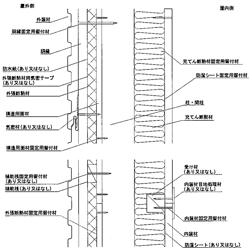
鉛直断面図
