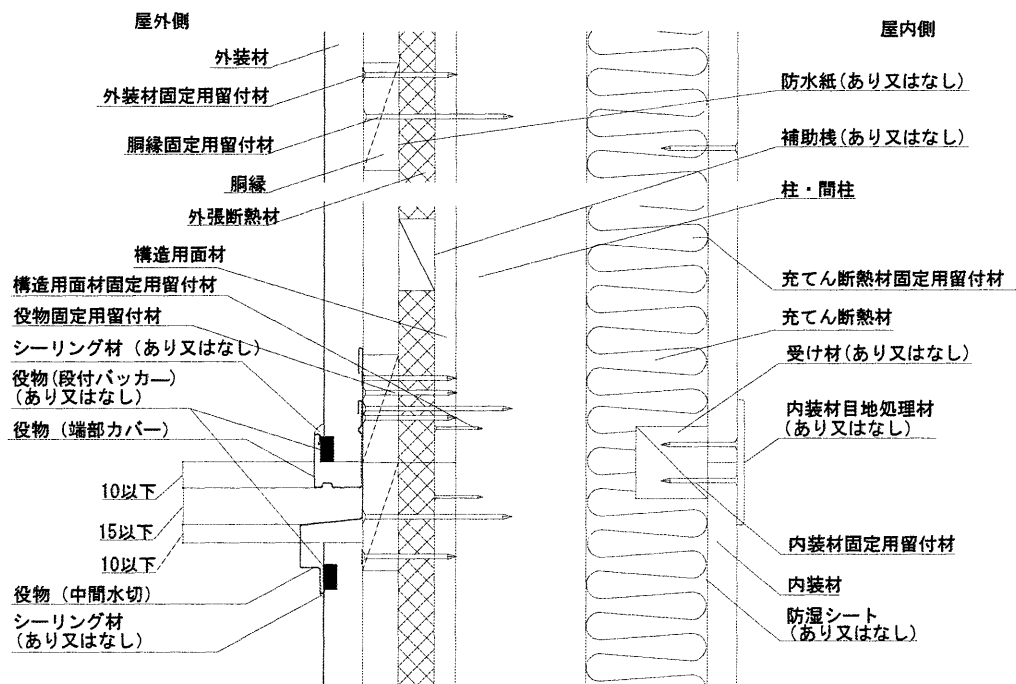
鉛直断面図
