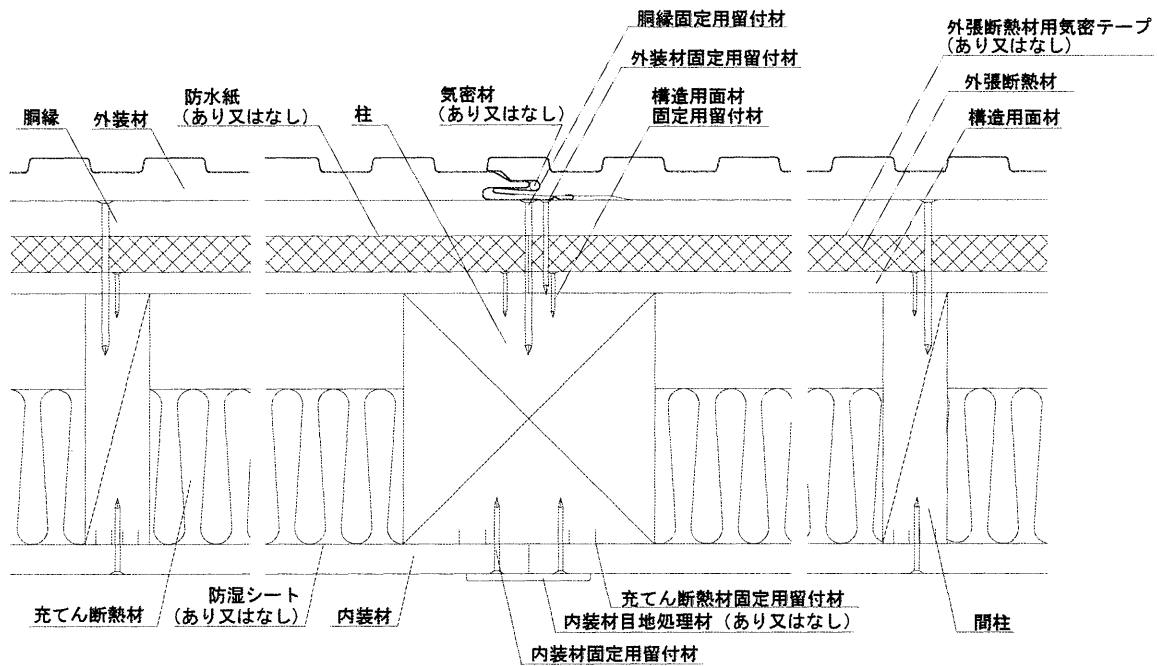
水平断面図
