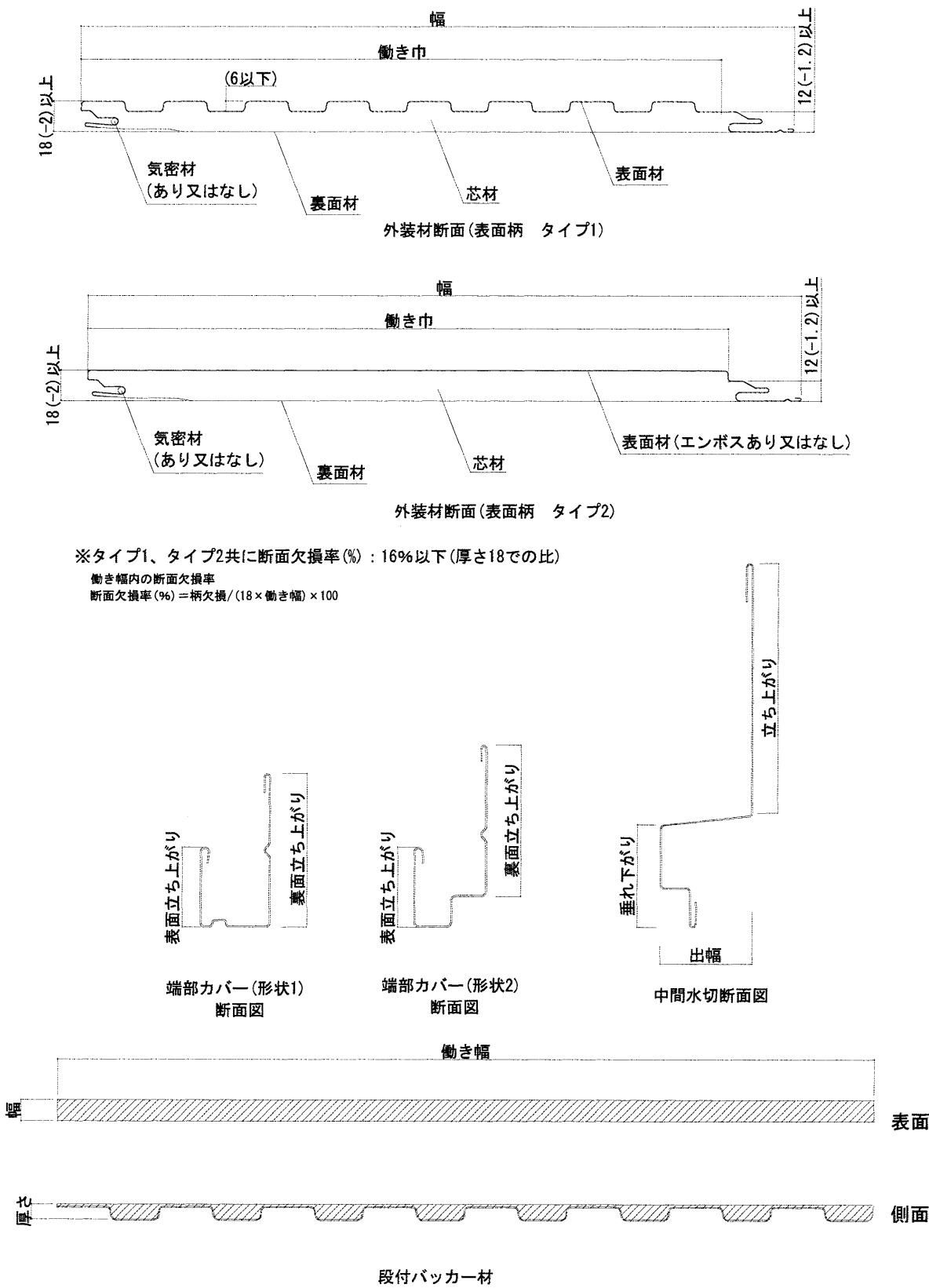
図3 構造説明図
