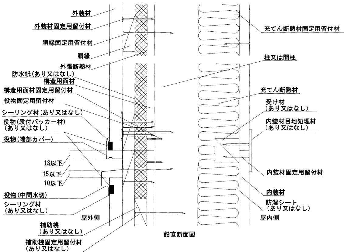
図2 構造説明図 (充てん断熱材あり)
