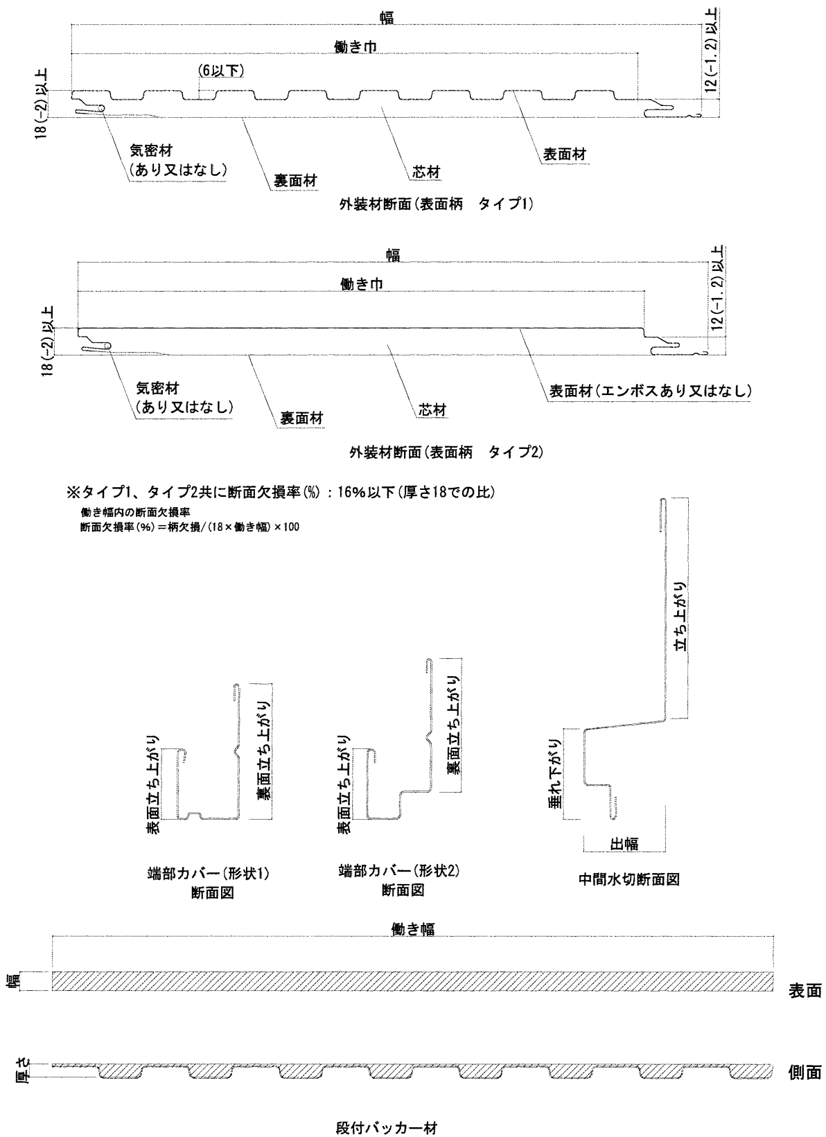
図3 構造説明図 (充てん断熱材)
