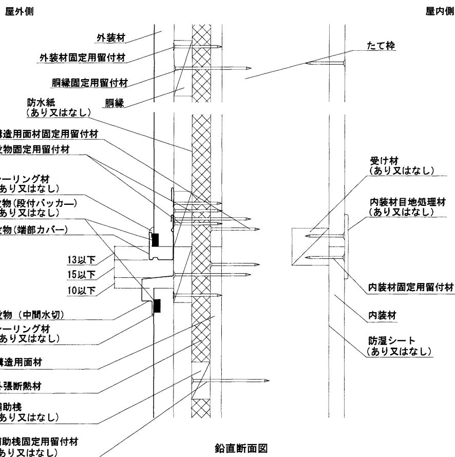
図2 構造説明図 (充てん断熱材なし)
