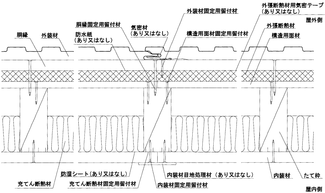
水平断面図
