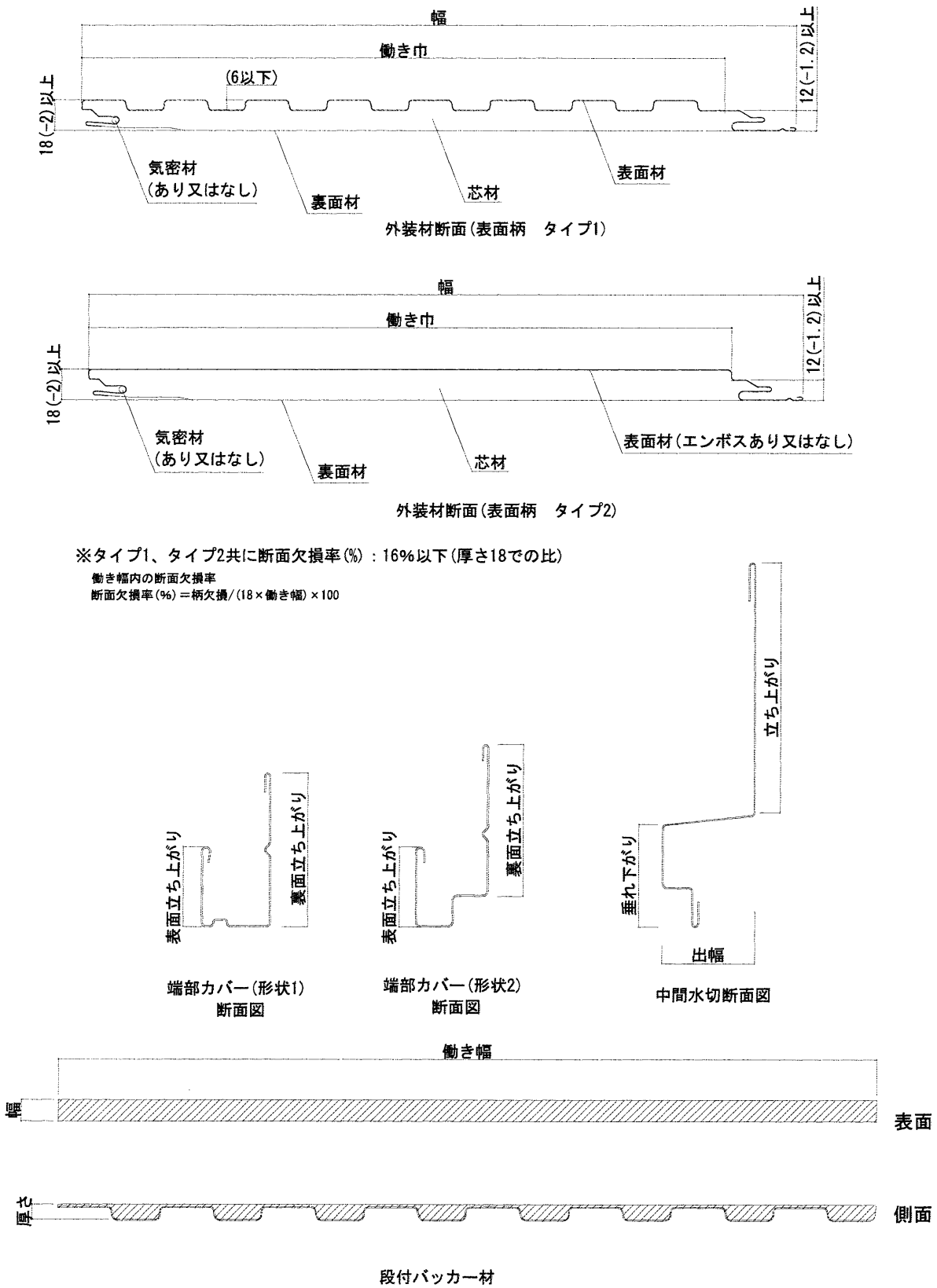
図3 構造説明図
