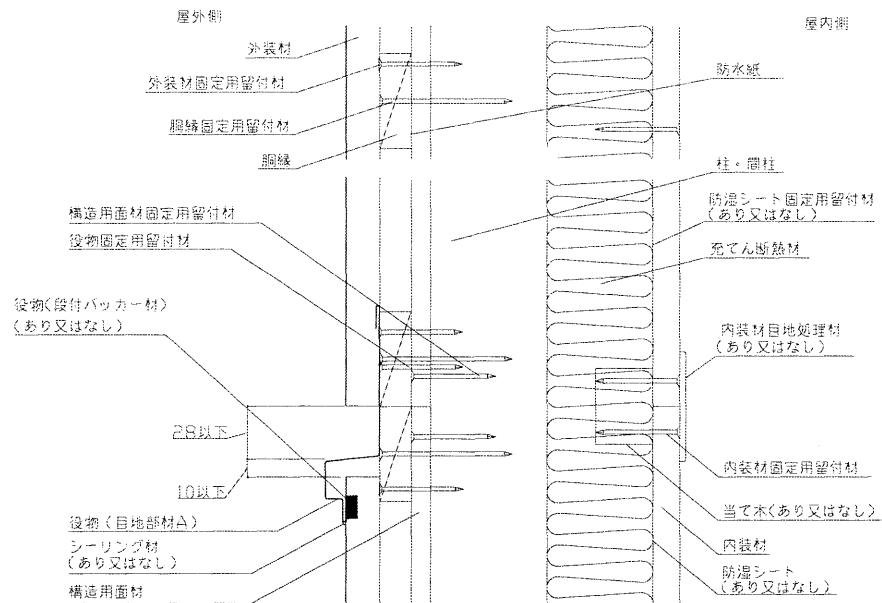
垂直断面図
