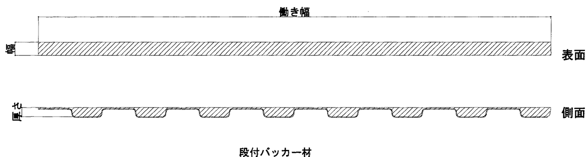
図7 構造説明図
