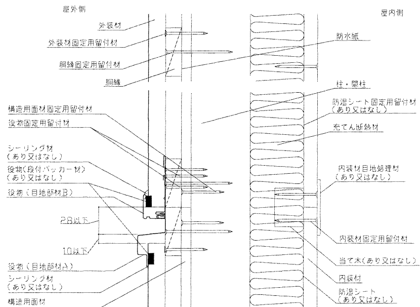
垂直断面図
