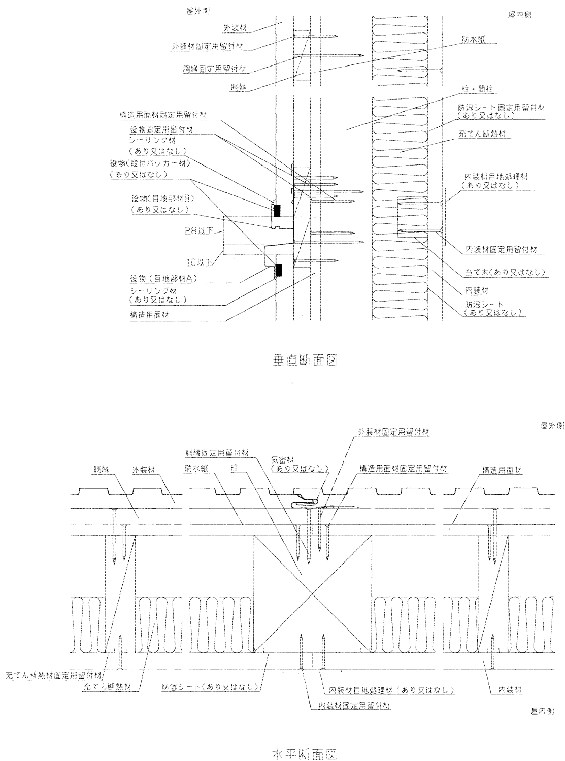
図6 構造説明図
