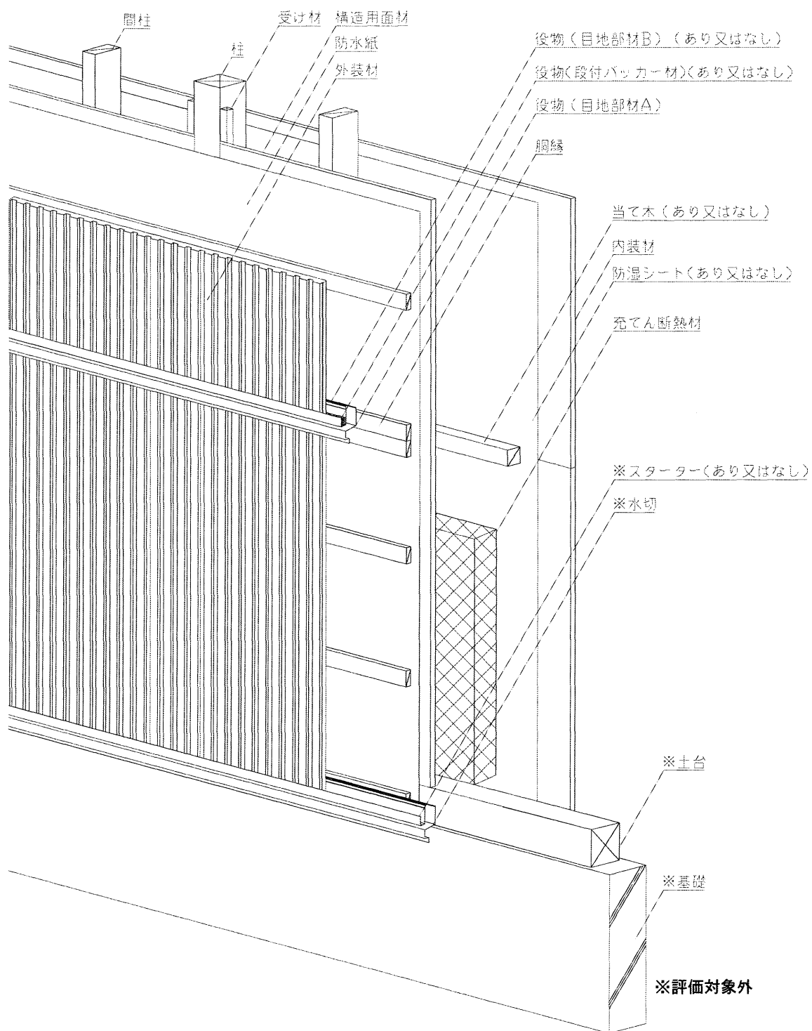
図1 構造説明図
