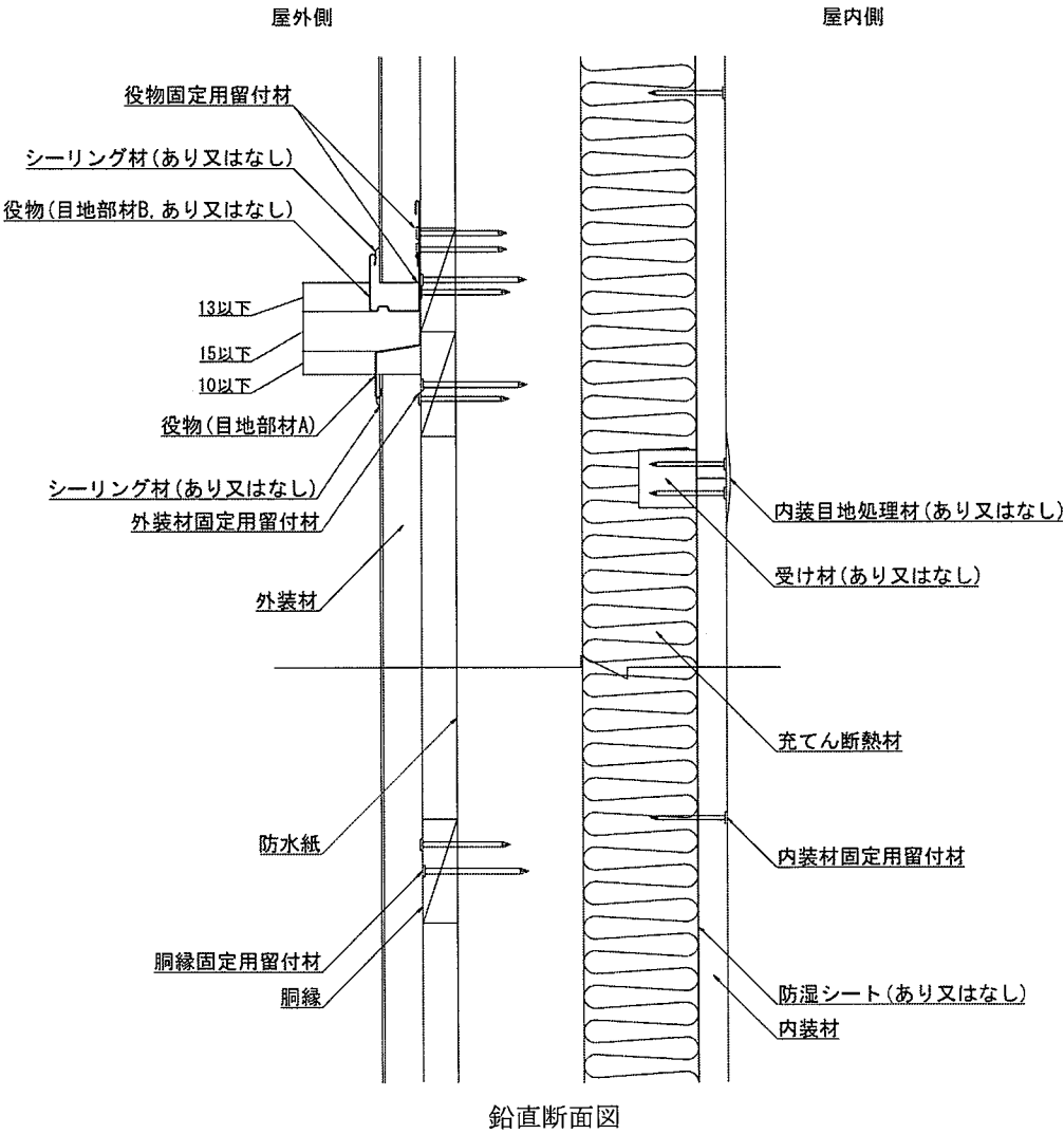
図2 構造説明図
