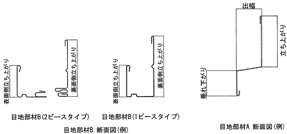
図3 構造説明図
