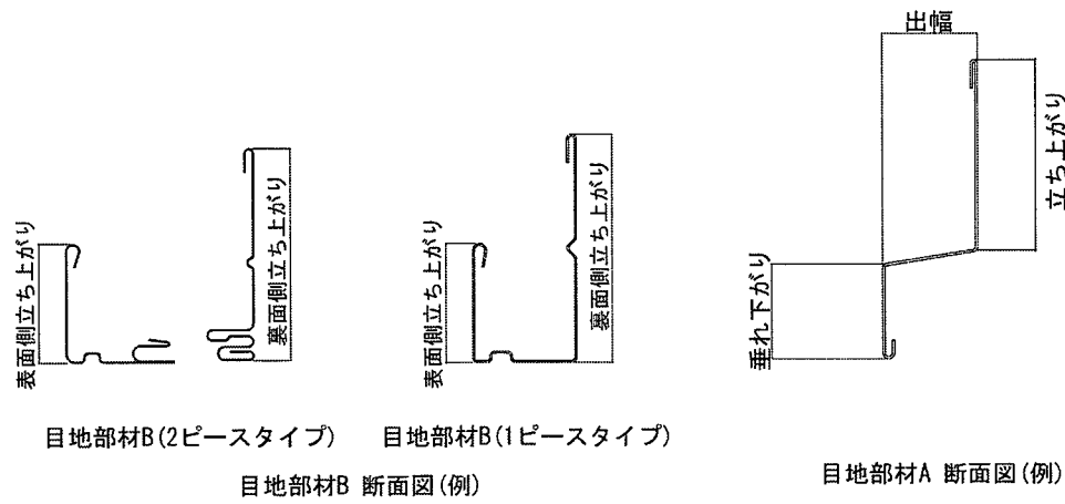
図3 構造説明図
