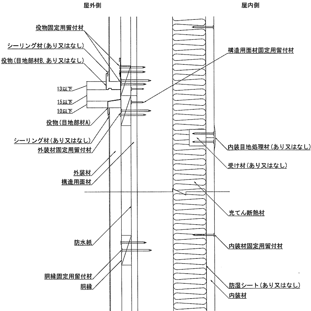
鉛直断面図
