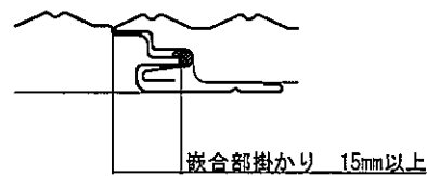
嵌合部詳細
