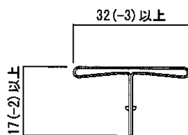
目地力バー(鋼板製)
