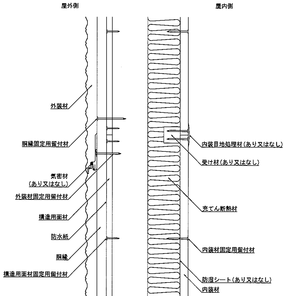
構造用面材あり 図 2 構造説明図
