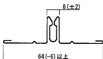
目地受け(鋼板製)
