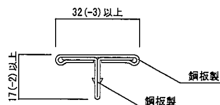
目地力バー(鋼板製)
