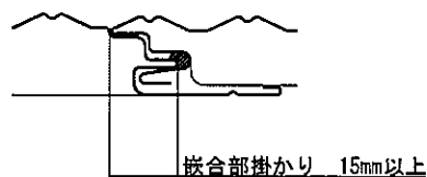
嵌合部詳細
